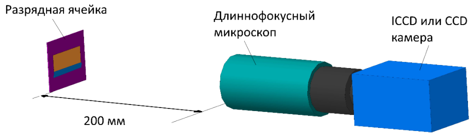
Рис. 2.12. Схема эксперимента с оптической регистрацией разряда
