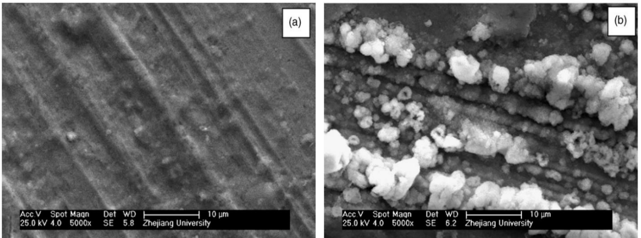
Рис. 1.31. Изображения поверхности медного образца (а) контрольного и (b) обработанного плазмой барьерного разряда [141].
