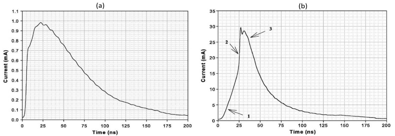
Рис. 1.15. Форма токовых импульсов положительной короны в воздухе атмосферного давления: (а) нерегулярный стример, U = 3.2 кВ ; (б) регулярный стример, U = 8.2 кВ [105].
