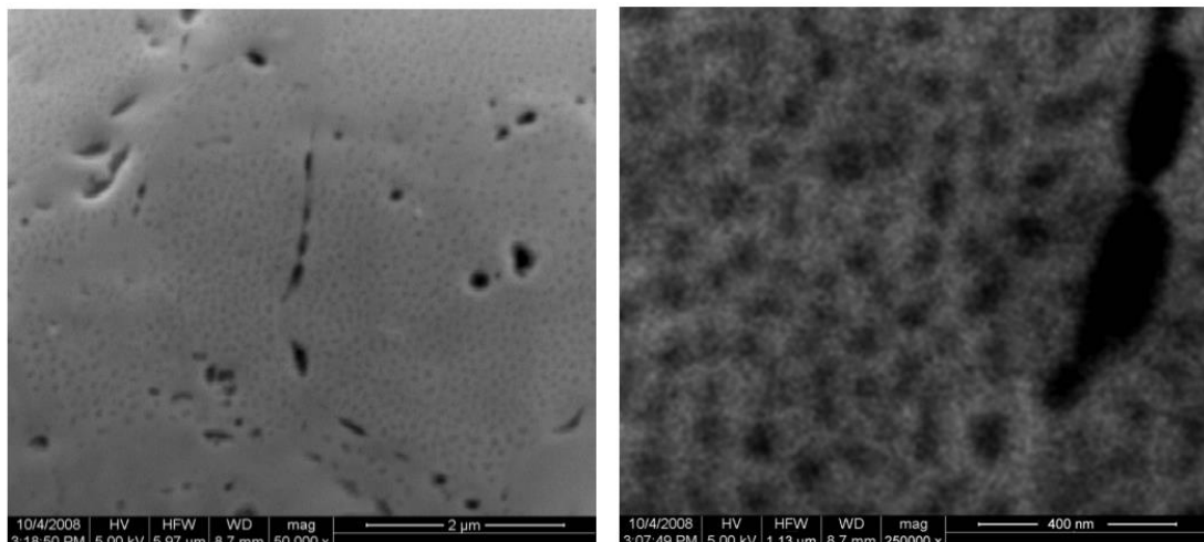
Рис. 1.26. Поверхность медного катода после воздействия на него отрицательного коронного разряда, существующего в режиме импульсов Тричела [136].
