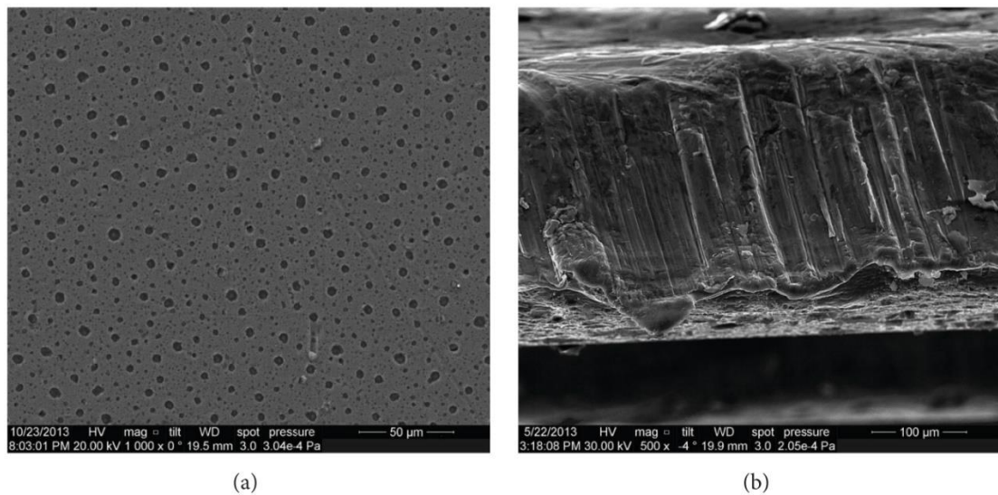
Рис. 1.27. Поверхность алюминиевого электрода после воздействия импульсной короны, покрытая пористым слоем оксида (a) и поперечный разрез такого электрода (b) [138].
