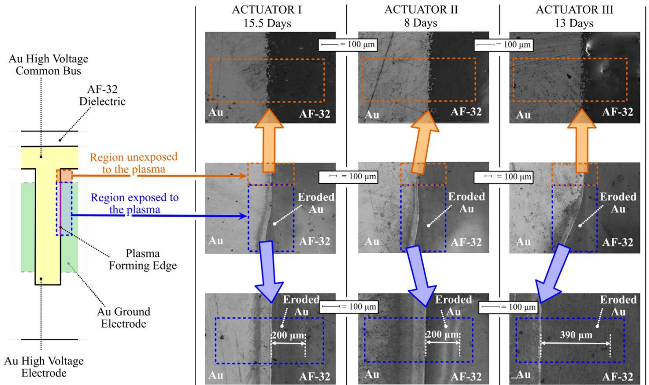
Рис. 1.35. Микроизображения кромок открытого плазмообразующего электрода после использования. Рисунок слева показывает соответствующие микрофотографиям участки электродов [150].
