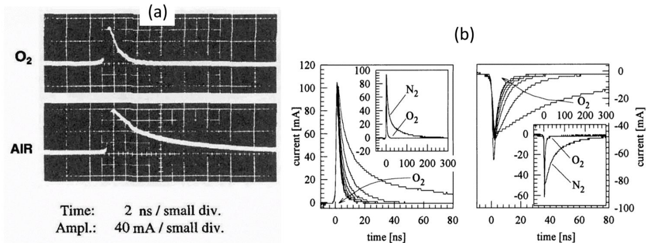
Рис. 1.17. Форма токовых импульсов, полученных в смесях O 2 -N 2 с различным содержанием O 2 (a) [5], (b) [37].
