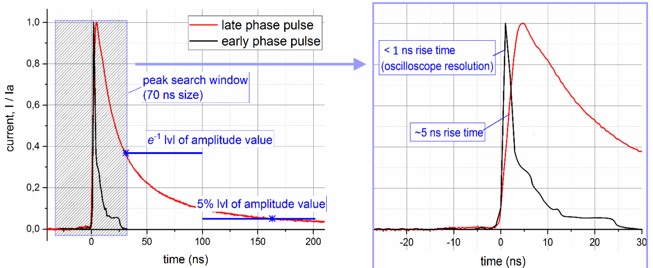
Рис. 4.10. Типичная форма нормализованных импульсов 2-ой группы для обработанного медного электрода до усреднения. Отрицательная полярность электрода. Черная линия - импульс ранней фазы, красная линия - длинный импульс, полученный на поздней фазе напряжения. Затененный прямоугольник показывает часть сигнала, анализируемую алгоритмом поиска импульсов.
