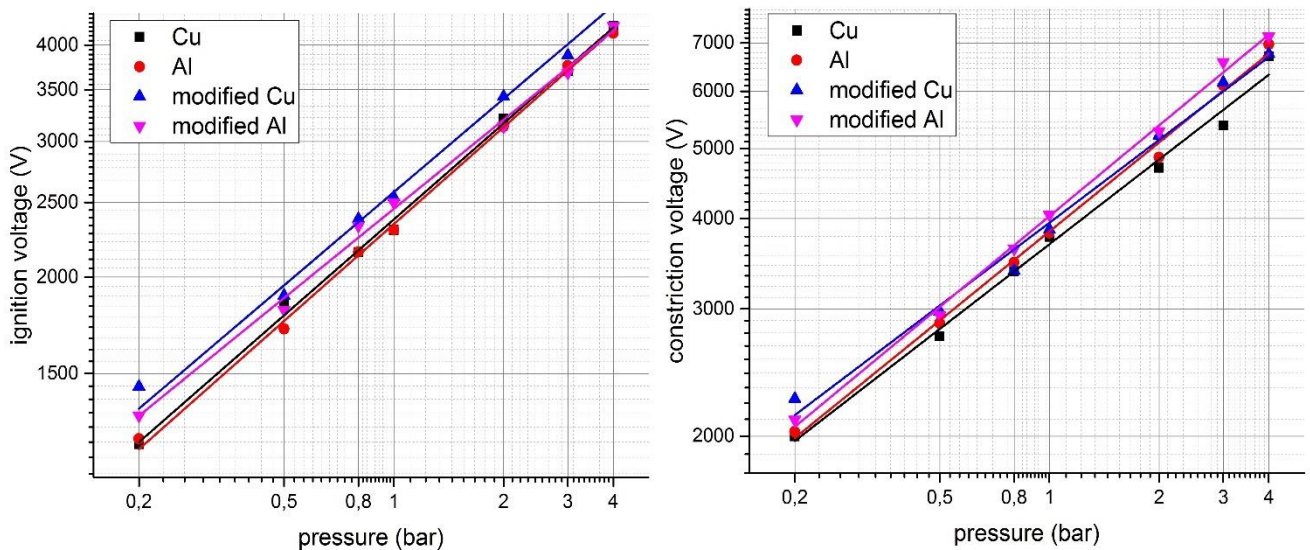
Рис. 3.16. Зависимости порогов зажигания (слева) и контракции (справа) от давления для различных типов коронирующих электродов.
