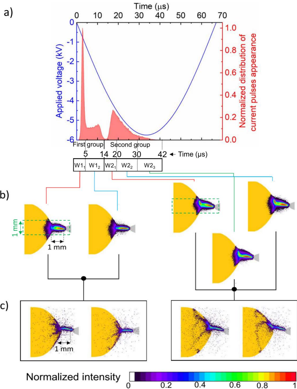
Рис. 1.20. (a) Гистограммы перенесенного за отрицательный полупериод заряда; (b) осредненные ICCD изображения микрозарядов, соответствующих различным областям гистограммы; (c) ICCD изображения МР без осреднения [110].
