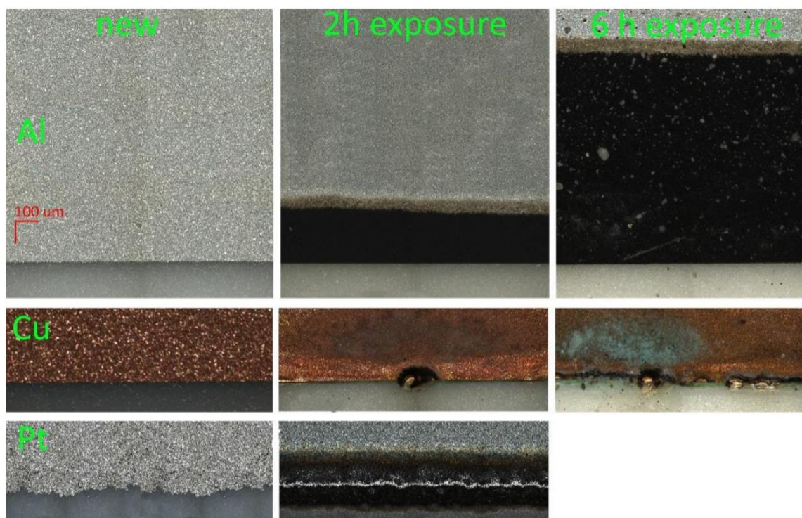
Рис. 3.13. Изображения кромок напыленных электродов
