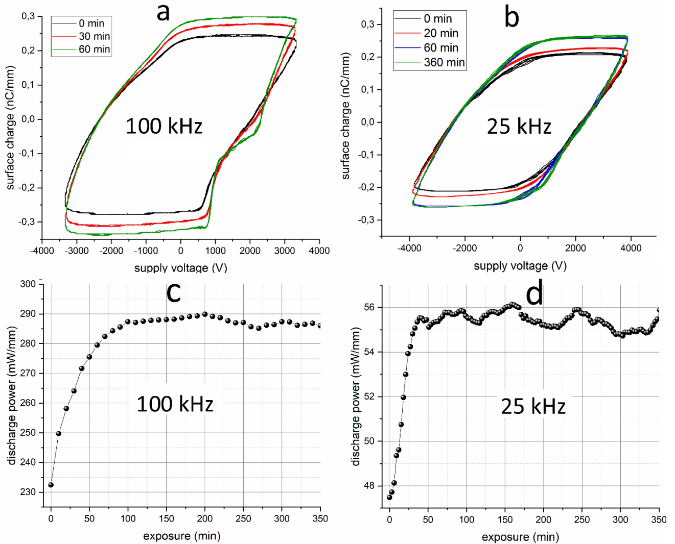
Рис. 3.11. (а), (б) ВКХ разряда в разные моменты времени для частот питающего напряжения 100 кГц и 25 кГц, соответственно. (с), (д) – Эволюция разрядной мощности для 100 кГц и 25 кГц. Электрод изготовлен из медной фольги.
