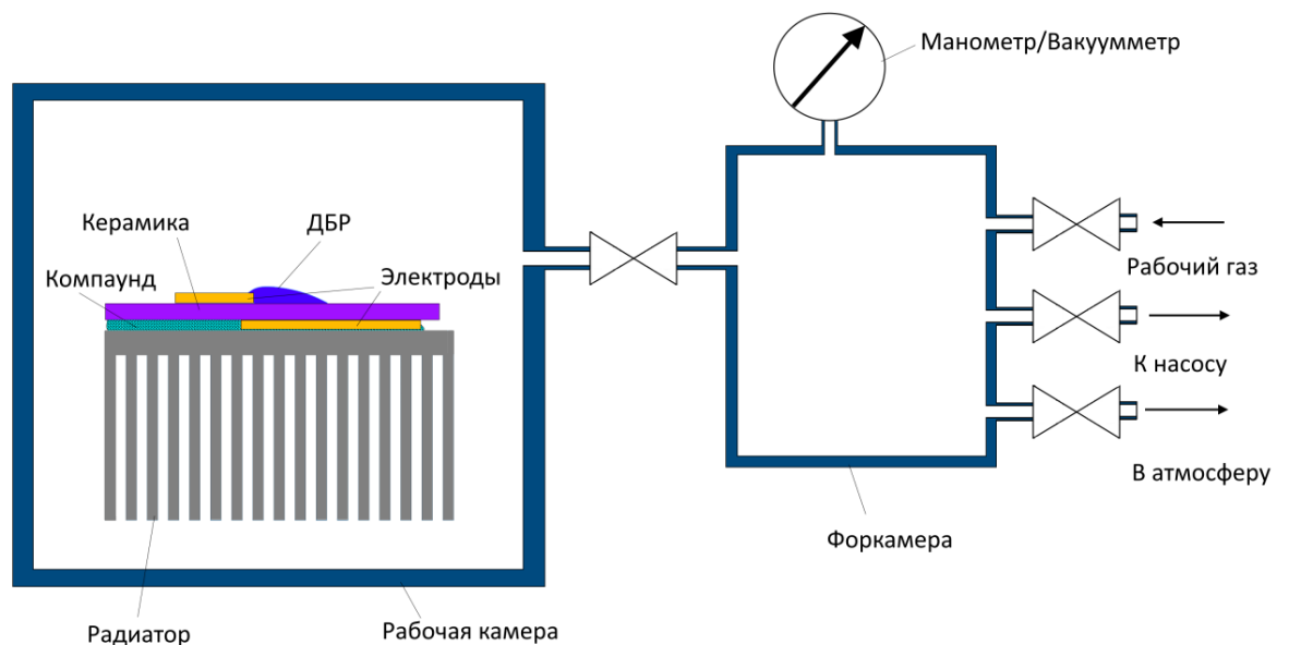
Рис. 2.13. Газовый стенд
