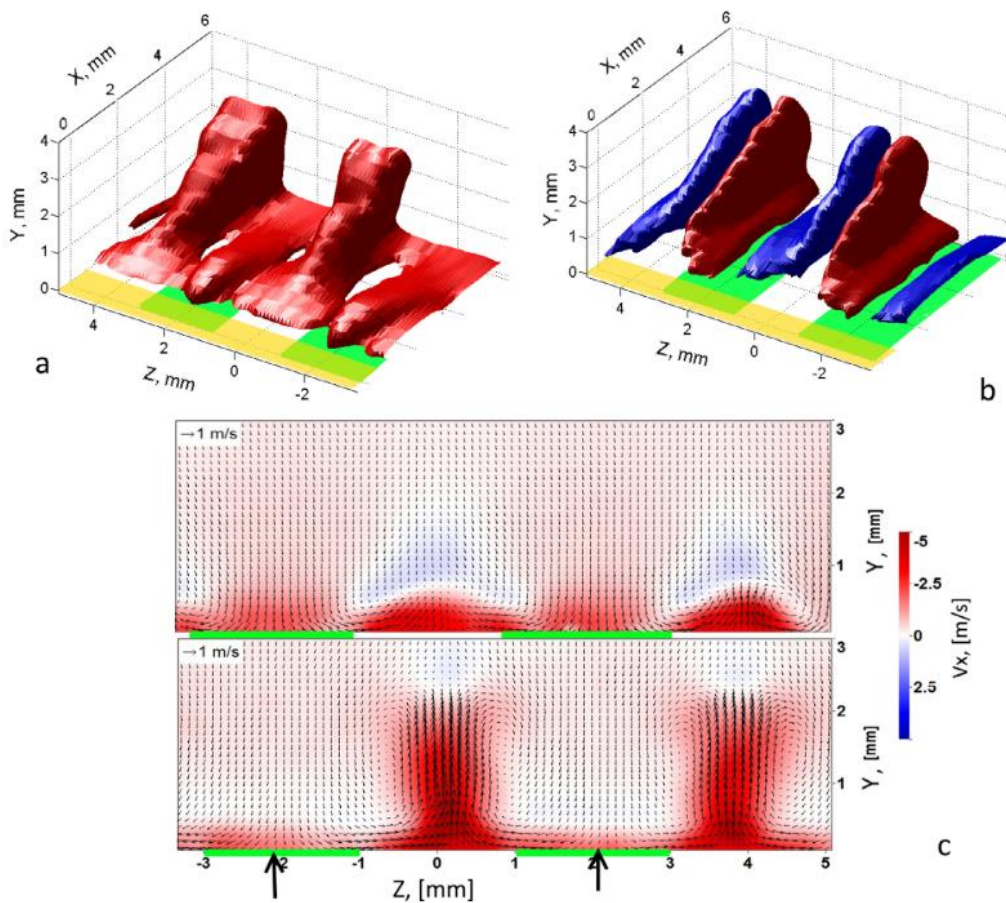
Рис. 5.3. Поля скорости индуцированного контрагированным ДБР течения в сечениях: (а) Исоповерхность скорости пристенной струи u = 1 \text{ м / с} , (б) Исоповерхность X компоненты завихренности \omega_x = \pm 10^3 \text{ 1 / с} . (с) Поперечные сечения поля потока при X = 1 \text{ мм} , X = 3.5 \text{ мм} .
