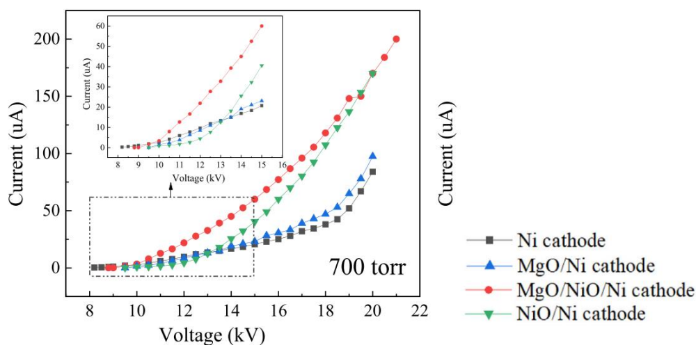
Рис. 1.25. Вольт-амперные характеристики разрядов постоянного тока с различными катодами в азоте при давлении 700 Торр [129].
