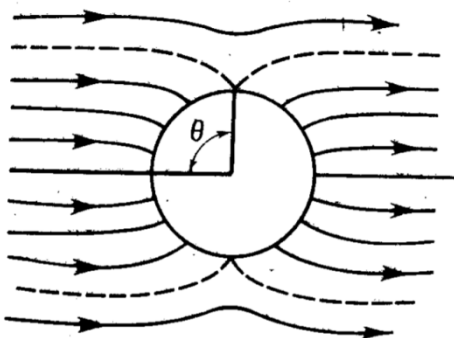
Рис. 2.19. Частица в электрическом поле.
