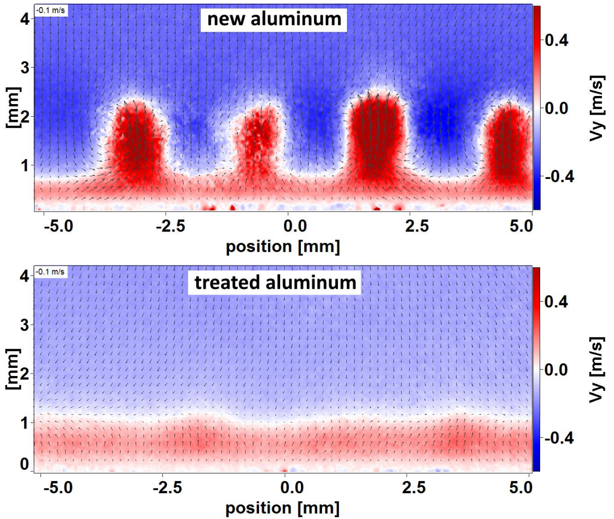
Рис. 5.4. Поля скорости течений в перпендикулярной развитию разряда плоскости на расстоянии 7 мм от алюминиевой коронирующей кромки
