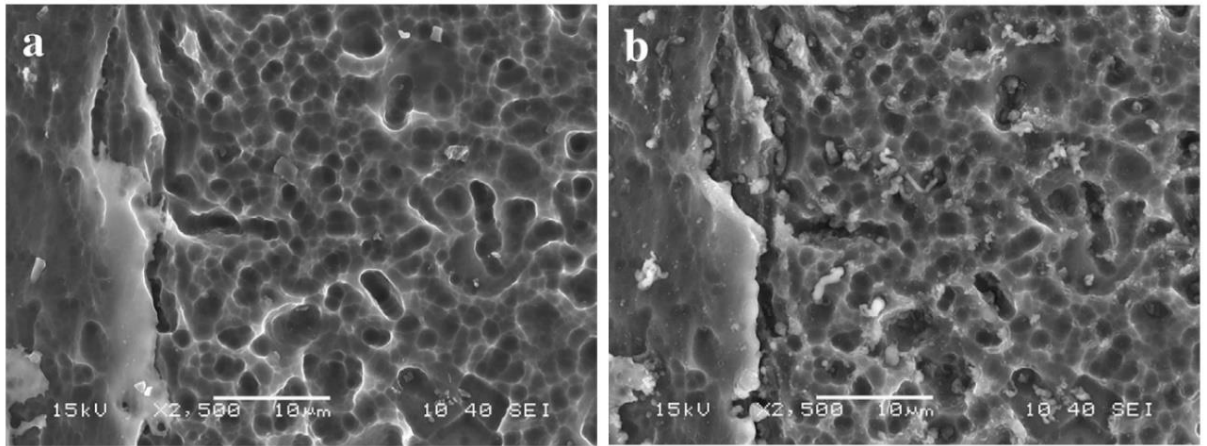
Рис. 1.29. (a) поверхность алюминия с дефектами, вызванными щелочным травлением (b) результат обработки поверхности объемным барьерным разрядом [139].
