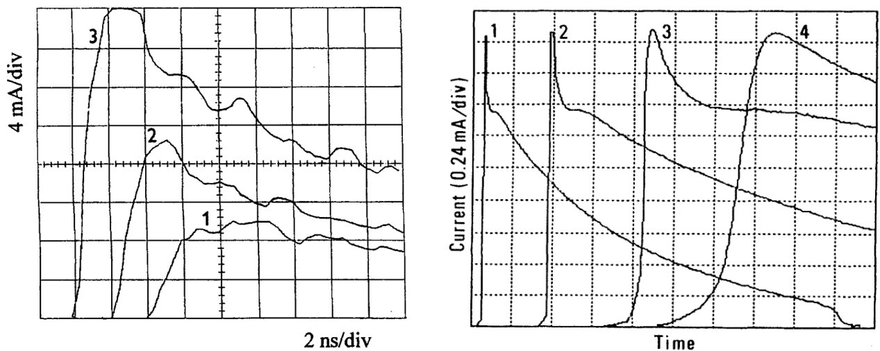
Рис. 1.11. (Слева) Форма импульсов Тричела коронного разряда, инициируемого в воздухе атмосферного давления при различных потенциалах коронирующего острия: (1) – 9.0 кВ (2) – 9.9 кВ (3) – 10.8 кВ [96]; (справа) форма импульсов Тричела коронного разряда, инициируемого в СО при давлении 0.13 бар с разными временными развертками: (1) 0.5 мкс/дел (2) 0.2 мкс/дел, (3) 50 нс/дел, (4) 10 нс/дел [97].
