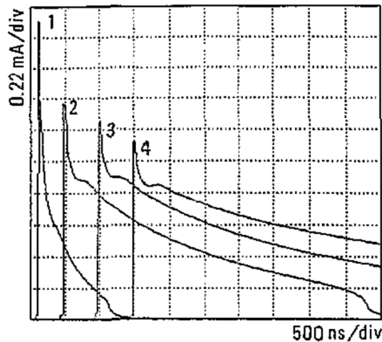
Рис. 1.13. Осциллограммы импульсов Тричела в смесях N 2 -O 2 : 1) N 2 + 40% O 2 ; 2) N 2 + 20% O 2 ; 3) N 2 + 10% O 2 ; 4) N 2 + 5% O 2 . P = 13.3 кПа и U = 3.1 кВ [102].
