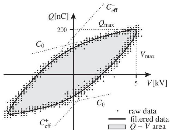
Рис. 2.7. Вольт-кулонная циклограмма пДБР [154].
