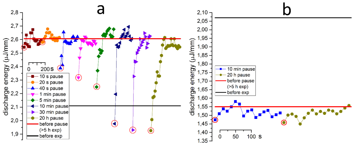
Рис. 3.12. Динамика мощности разряда после паузы в работе разряда для медного (а) и алюминиевого (б) электродов. Красными кружками отмечены моменты возникновения разряда после паузы. Красная линия обозначает энергию разряда до паузы, черная линия - начальная энергия разряда (до модификации)
