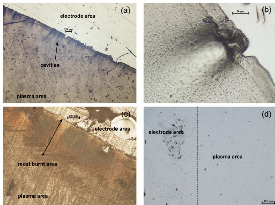
Рис. 1.32. Рельеф поверхности диэлектрических барьеров после воздействия пДБР с амплитудой 18 кВ в течение 10 минут: (а), (b) – оргстекло, (с) ПВХ, (d) боросиликатное стекло. [145]
