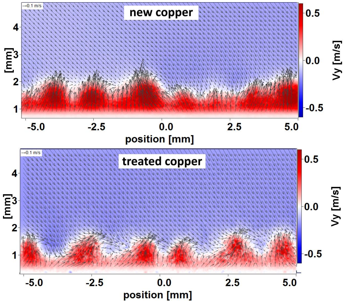
Рис. 5.5. Поля скорости течений в перпендикулярной развитию разряда плоскости в случае медного электрода
