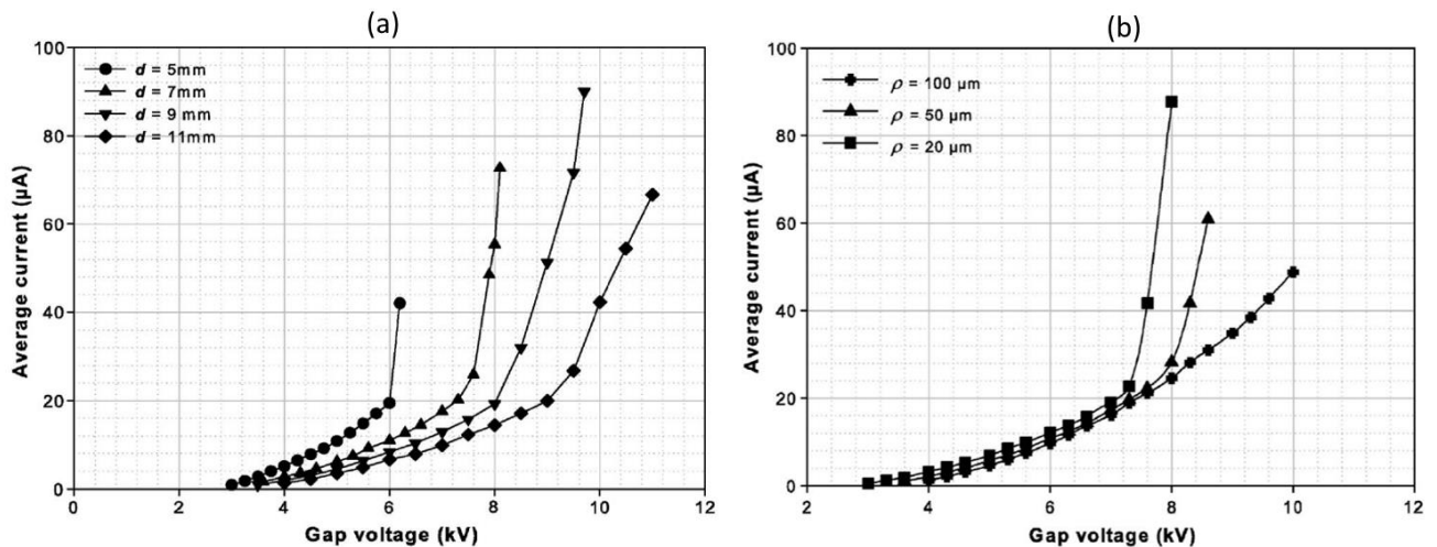
Рис. 1.16. Зависимость среднего тока стримеров приложенного к электродам напряжения (а) при различных межэлектродных расстояниях , (б) при различных радиусах кривизны анода [105].
