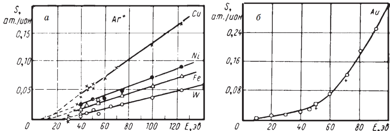
Рис. 1.23. Зависимость коэффициента распыления различных материалов от энергии бомбардирующих катод атомов аргона [114].
