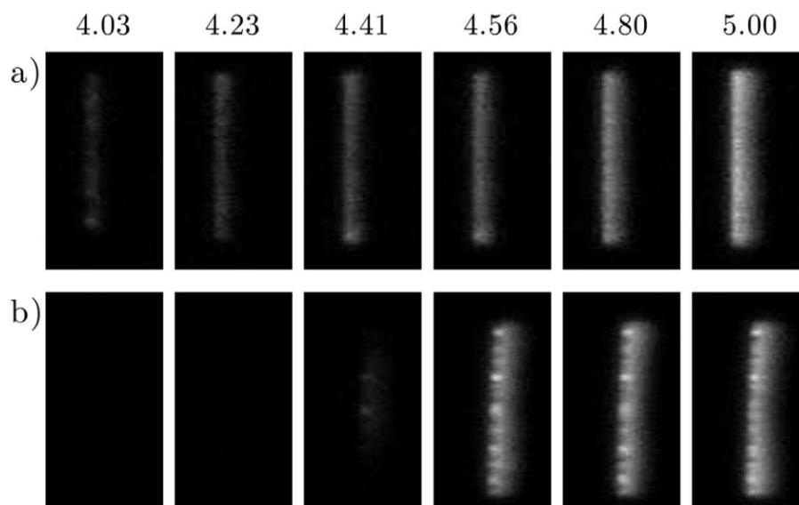
Рис. 1.37. Разряд в системах с вольфрамовыми электродами (а) и медными электродами (б). Размах приложенного напряжения указан над каждым столбцом изображения в кВ. [151].
