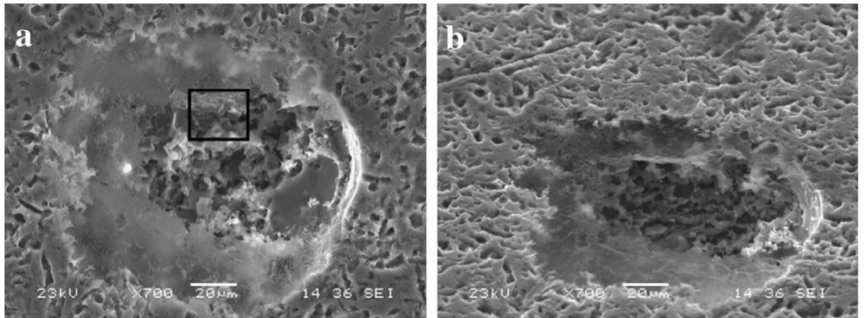
Рис. 1.30. Изображения кратеров на оксидном слое на образце, обработанном барьерным разрядом в атмосферном воздухе в течение 20 минут [139].
