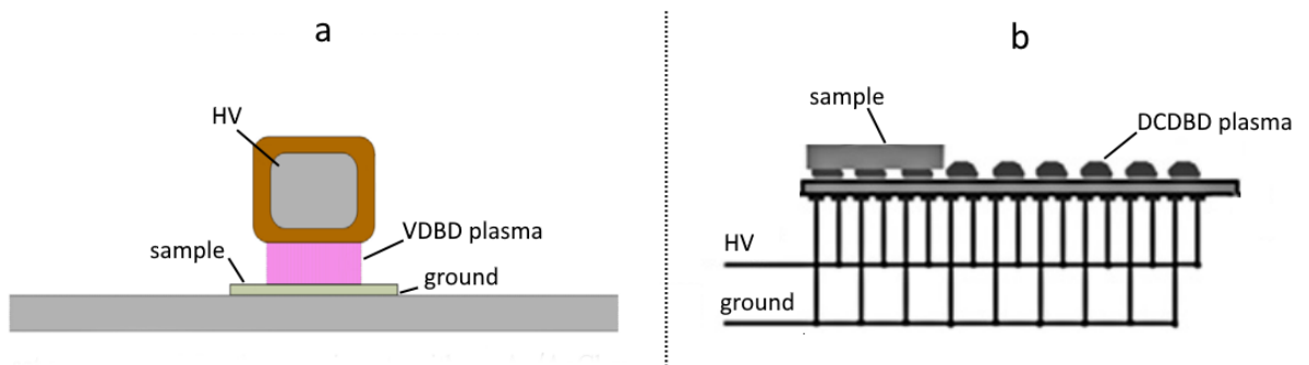
Рис. 1.28. Конфигурации электродов, используемые для обработки поверхностей плазмой барьерного разряда: а) обработка поверхности объемным ДБР [139] , б) обработка поверхности с помощью диффузного компланарного ДБР [140].
