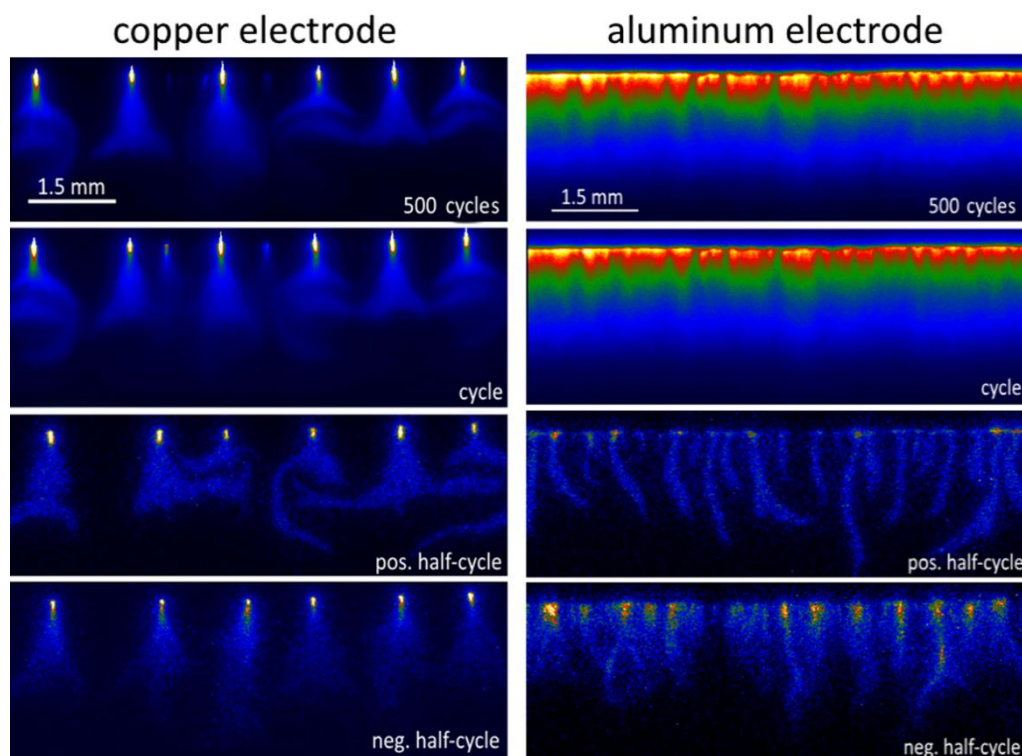
Рис. 4.1. Интегральные изображения разряда в случае алюминиевого и медного электродов, модифицированных плазмой пДБР. Снимки были сделаны с разной экспозицией (вверх-вниз) - 500 периодов питающих напряжений, 1 период, положительный и отрицательный полупериод.
