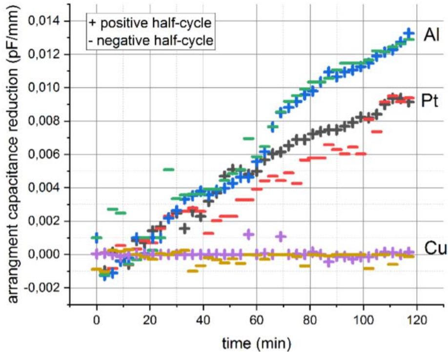
Рис. 3.15. Снижение емкости электродных систем, посчитанное в «темных» фазах питающего напряжения
