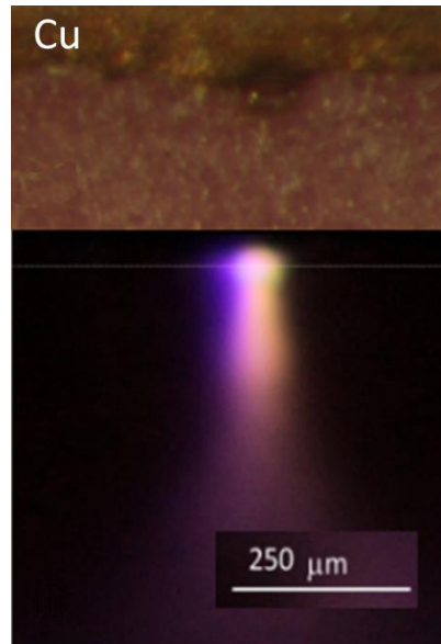
Рис. 3.17. Изображение медной кромки и микроразрядного канала, полученные с экспозициями, существенно превышающими период питающего напряжения
