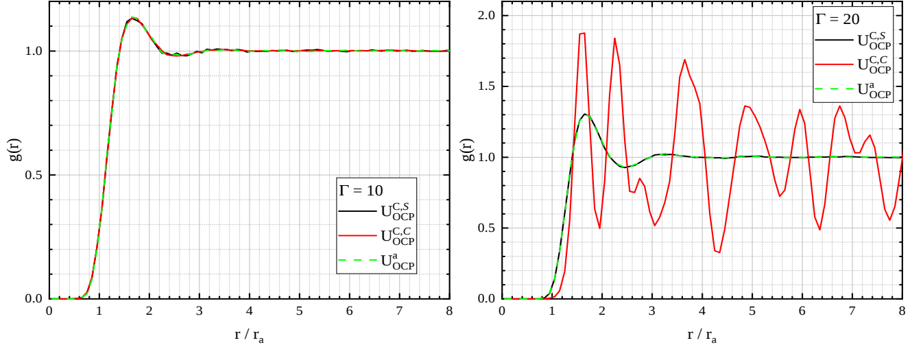
Рис. 4.8. Парные корреляционные функции ОКП для различных потенциалов взаимодействия при \Gamma = 10 (слева) и \Gamma = 20 (справа) для N = 10^3 . Черной сплошной и зеленой пунктирной линиями показаны результаты для кулоновского потенциала в сферической области (1.246) и УУПЭ (1.248) соответственно, а красной линией для кулоновского потенциала в кубической области (1.247).
