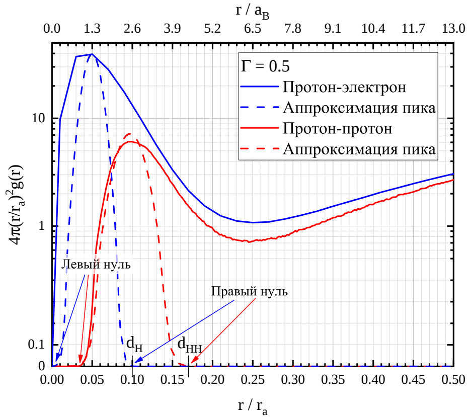
Рис. 3.6. Иллюстрация алгоритма выбора расстояний d_H и d_{HH} . Синей и красной сплошной линией показаны 4\pi r^2 g(r) в случае электрон-протон и протон-протон соответственно. Для наглядности процедуры пунктирными линиями изображены положения пиков в Гауссовой форме; при этом совпадение пунктирной линии и сплошной не требуется. В данном случае, «правый нуль» относится к пунктирным линиям.
