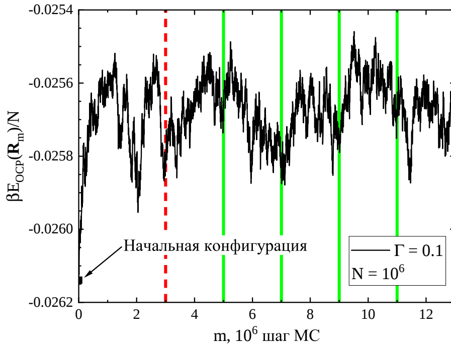
Рис. 3.4. Характерное поведение энергии при моделировании. В данном случае, представлена зависимость потенциальной энергии ОКП \beta E_{\text{ОСР}}^a/N для 10^6 частиц при \Gamma = 0.1 в моделировании МК. Вертикальная пунктирная красная линия обозначает начало равновесного участка. Зелёные сплошные вертикальные линии показывают разбиение равновесного участка на блоки. Зависимость энергии в моделировании методом МД имеет схожий вид.
