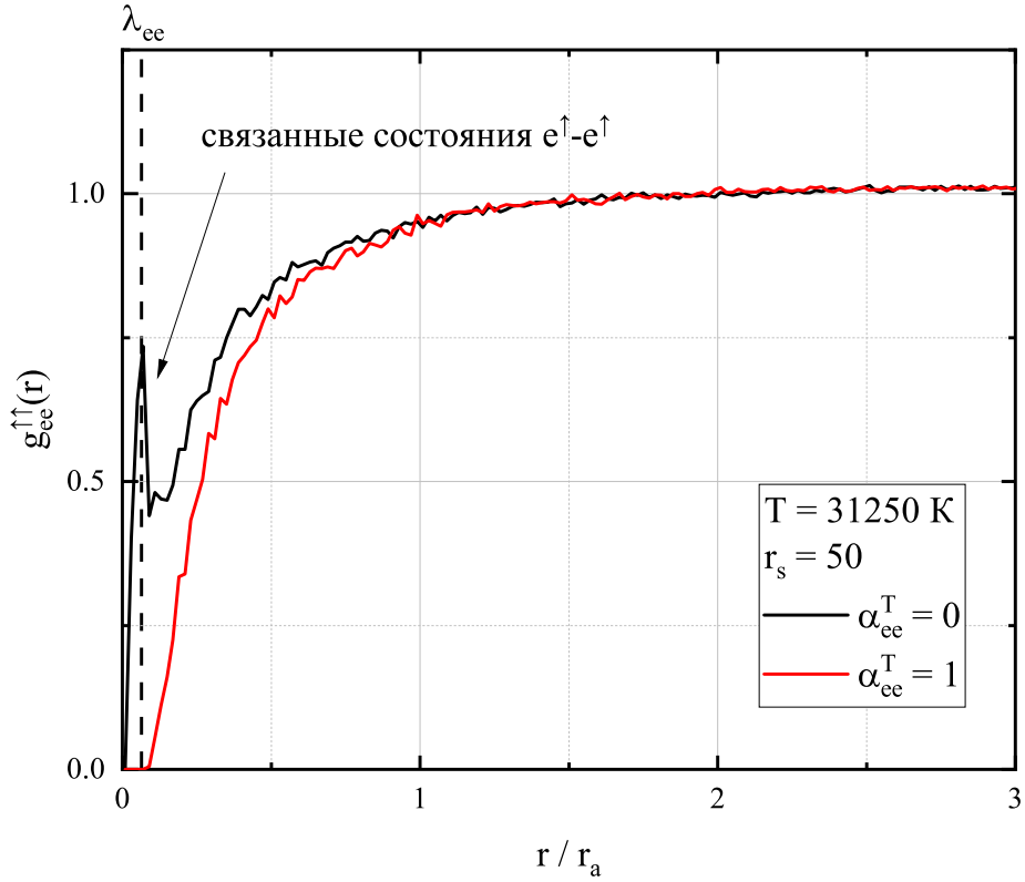
Рис. 2.3. Пример образования связанных состояний электронов с одинаковой проекцией спина. Черная кривая получена без модификации сил ( \alpha_{ee}^T = 0 ), а красная с использованием (2.94) с параметром \alpha_{ee}^T = 1 .
