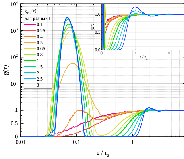
(а) РФР g_{p-p}(r) между всеми протонами в системе.
