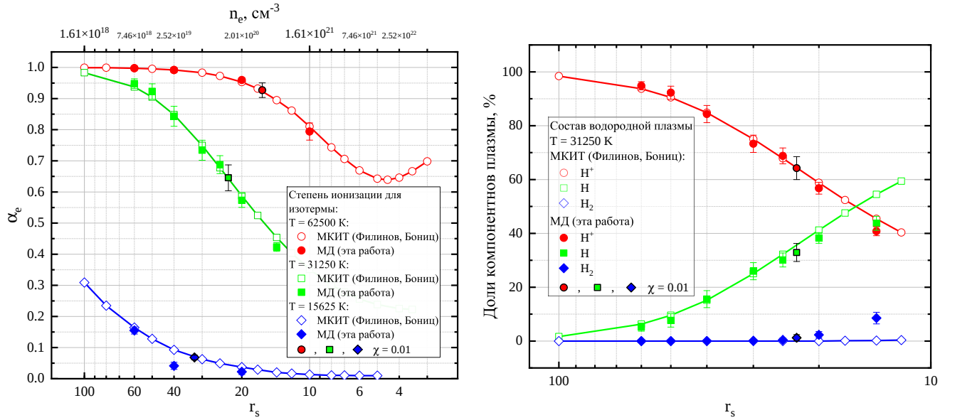
(а) Степень ионизации в зависимости от параметра r_s на трех изотермах: T = 62500 \text{ K} , T = 31250 \text{ K} и T = 15625 \text{ K} . Пустыми символами показаны данные из рис. 23 работы [114], который был получен на основании данных моделирования [211]. Закрашенными символами показаны данные МД, полученные в этой работе. Закрашенные символы с черной каемкой показывают значение при \chi = 0.01 ; слева от такого символа \chi < 0.01 , справа — \chi > 0.01 .
