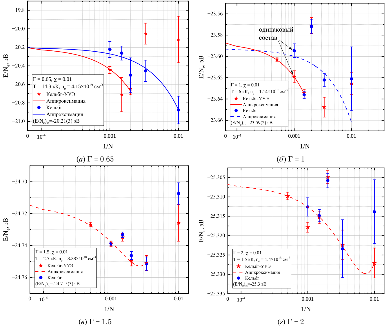
Рис. 5.11. Зависимость полной энергии на один электрон невырожденной водородной плазмы от обратного числа частиц в области 0.65 \leq \Gamma \leq 2 при \chi = 0.01 . По горизонтальной оси в промежутке (10^{-4}, 0.014) используется логарифмический масштаб; при 1/N < 10^{-4} используется линейный масштаб. Хорошо видно, что при сильной неидеальности зависимость от числа частиц является скачкообразной, из-за чего получить надежный термодинамический предел не представляется возможным при использовании N \leq 10^3 .
