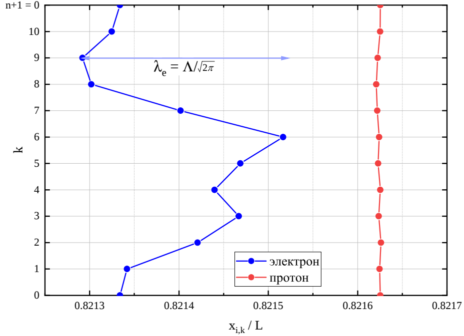
Рис. 2.2. Представление электронов и протонов в виде интегралов по траекториям для n = 10 . Горизонтальная ось показывает проекцию x -ой координаты частицы \mathbf{r}_{i,k} = (x_{i,k}, y_{i,k}, z_{i,k}) , а вертикальная ось показывает номер высокотемпературного разбиения или «бусины», k . Каждая траектория замкнута; то есть \mathbf{r}_{i,n+1} = \mathbf{r}_{i,0} . Характерный размер электрона равен \lambda_e = \sqrt{\hbar^2 \beta / m_e} = \Lambda / \sqrt{2\pi} , а характерный размер протона равен \lambda_p = \sqrt{\hbar^2 \beta / m_p} \ll \lambda_e ( \lambda_p меньше \lambda_e в \sqrt{m_p / m_e} \approx 43 раза).
