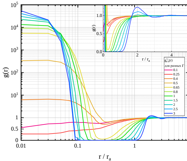
(в) РФР g_{e-e}^{\uparrow\downarrow}(r) между всеми электронами с различной проекцией спина в системе.
