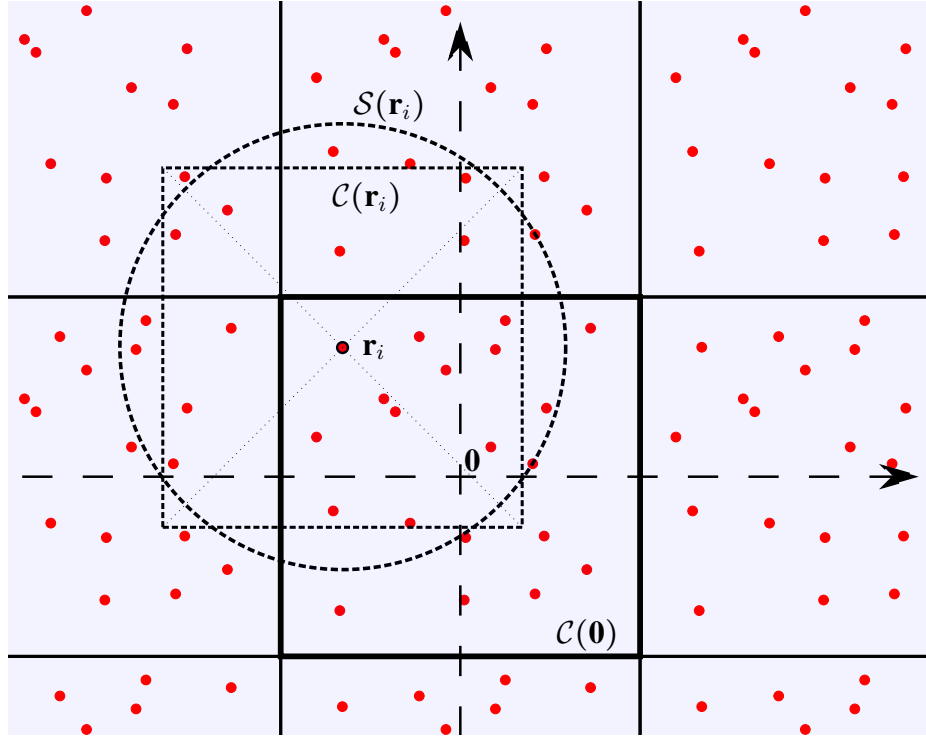
Рис. 1.4. Иллюстрация процедуры расчета потенциала \phi(\mathbf{r}_i) в точке \mathbf{r}_i . В данном случае \mathbf{r}_i представляет собой положение иона в верхнем левом углу основной ячейки, а \mathbf{0} обозначает начало координат. Для вычисления потенциала сначала определяется кубическая C(\mathbf{r}_i) (или сферическая S(\mathbf{r}_i) ) область, центрированная в точке \mathbf{r}_i . Объем этой области составляет V = L^3 ( V = 4\pi r_m^3/3 , где r_m = (4\pi/3)^{-1/3}L ). Затем выполняется интегрирование по этой области (см. уравнение (1.89)). Учитываются все взаимодействия иона с другими частицами внутри области. Процедура интегрирования соответствует правилу БИ. Для упрощения иллюстрация приведена для двумерной системы. Границы основной ячейки выделены жирными линиями, а области интегрирования показаны пунктирными линиями.
