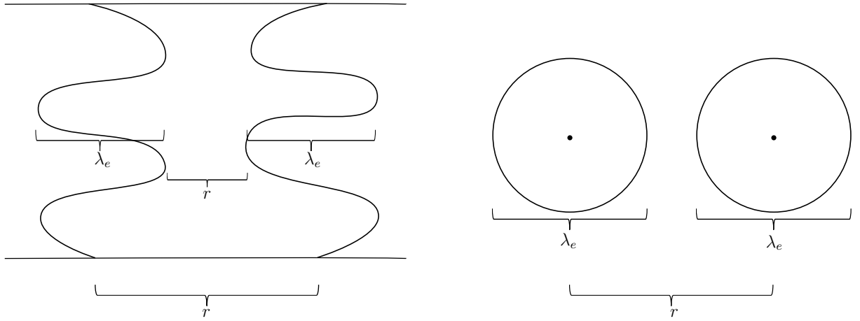
Рис. 2.4. Качественная иллюстрация способа учета конечного размера двух электронов в силах (слева по аналогии с рис. 2.2; справа качественно показаны две траектории на плоскости). Показаны характерные траектории двух электронов с одинаковой проекцией спина (перестановка тождественная). Размах каждой траектории равен \lambda_e . Центры этих траекторий находятся на расстоянии r , тогда как взаимодействие происходит между всеми точками траекторий, в том числе на расстоянии r - \lambda_e . Таким образом, отталкивание между электронами должно усилиться.
