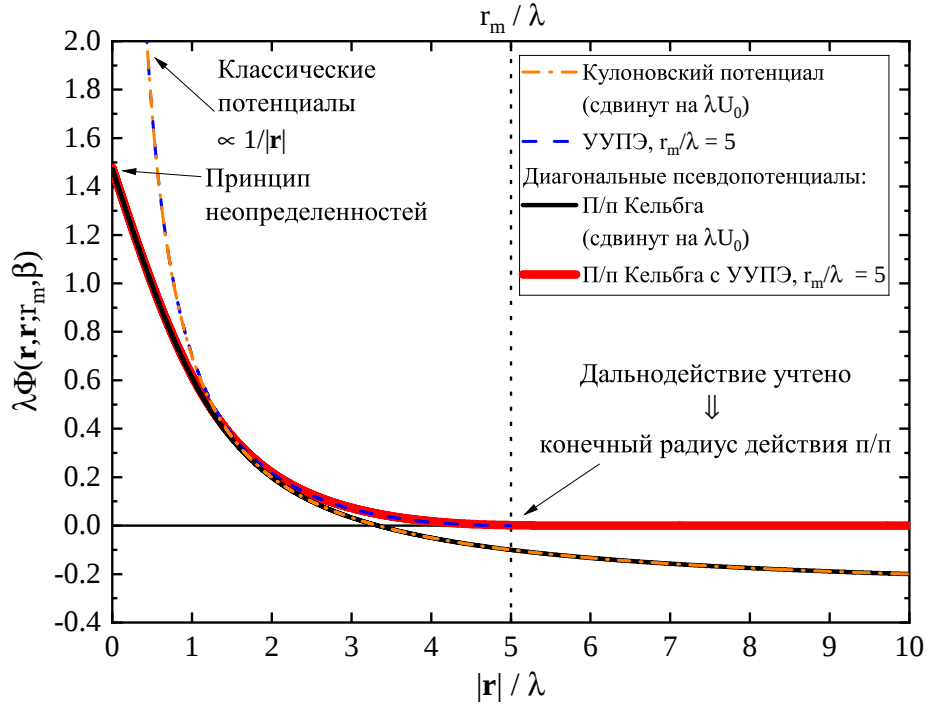
Рис. 2.1. Потенциалы и псевдопотенциалы взаимодействия для кулоновских систем. Индексы ij опущены. Классические потенциалы (кулоновский и УУПЭ) неограниченно возрастают при r \rightarrow 0 . Учет принципа неопределенности приводит к устранению этой расходимости и конечности псевдопотенциала при r \rightarrow 0 . На больших расстояниях r \gg \lambda квантовые эффекты практически не оказывают влияние, поэтому кулоновский потенциал и УУПЭ совпадают с псевдопотенциалом Кельбга и Кельбга-УУЭ соответственно. Учет эффектов дальнодействия в УУПЭ и Кельбг-УУЭ п/п приводит к конечному радиусу взаимодействия r_m , тогда как область взаимодействия кулоновского потенциала и псевдопотенциала Кельбга неограниченна. Кулоновский потенциал и псевдопотенциал Кельбга сдвинуты на величину \lambda U_0^a для удобства сравнения с п/п Кельбга-УУЭ; тем не менее, слагаемое U_0 не вносит вклад в потенциальную энергию в случаях кулоновского потенциала и исходного псевдопотенциала Кельбга.
