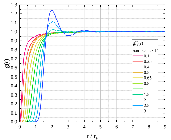
(г) РФР g_{e-e}^{\uparrow\uparrow}(r) между всеми электронами с одинаковой проекцией спина в системе.
