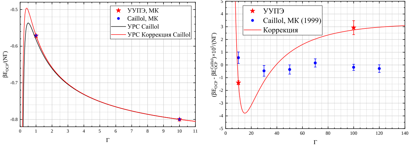
(а) Зависимость потенциальной энергии от параметра неидеальности.
