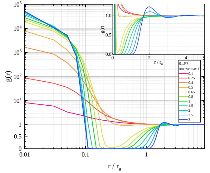
(б) РФР g_{p-e}(r) между всеми протонами и электронами в системе.
