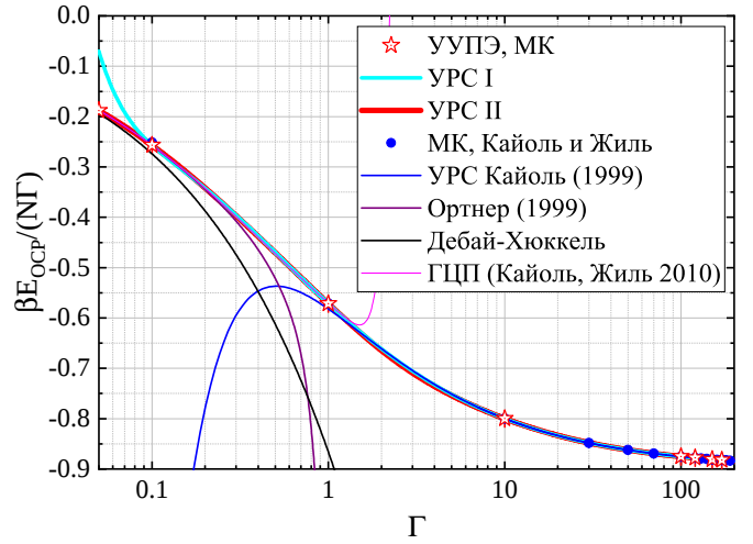
Рис. 8: Потенциальная энергия ОКП на частицу в зависимости от \Gamma . Красные звезды — данные МК из этой работы, синие точки — данные Кайоля, фиолетовая кривая — разложение Ортнера, черная — предел Дебая–Хюккеля.
