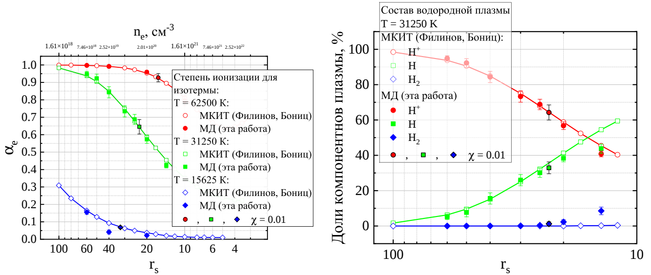
(а) Степень ионизации на трех изотермах.
