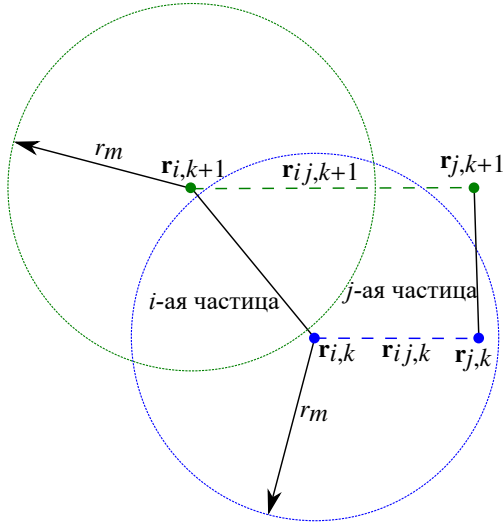
Рис. 4: Метод первого слоя: взаимодействие учитывается только для k -ых бусин.
