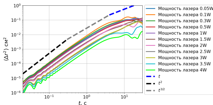
Рисунок 6. Среднеквадратичные смещения при мощности лазера от 4 Вт до 0.05 Вт.
