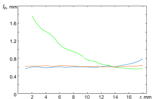
Рисунок 11. График зависимости радиального распределения среднего межчастичного расстояния в квазидвумерной структуре пылевых частиц в аргонной плазме (давление 5 Па) при различной мощности ВЧ разряда: синий график при W = 4.4 Вт; красный график при 6.9 Вт; зеленый график при 16.7 Вт.
