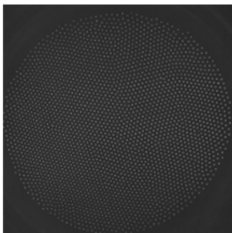
Рисунок 9. Кадр видеозаписи однородной монослойной структуры в плазме ВЧ разряда. W=6.9 Вт, P=5 Па
