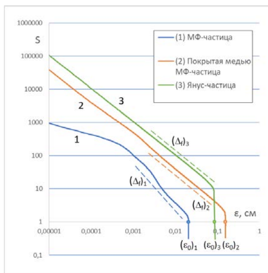
Рисунок 4. Динамическая энтропия первого пересечения для трех видов частиц при мощности лазера 1 Вт. Отмеченные пунктиром линии - логарифмические производные d(\lg(S(\epsilon)))/d(\lg \epsilon) . Точки на пересечении с осью абсцисс - величины областей локализации.
