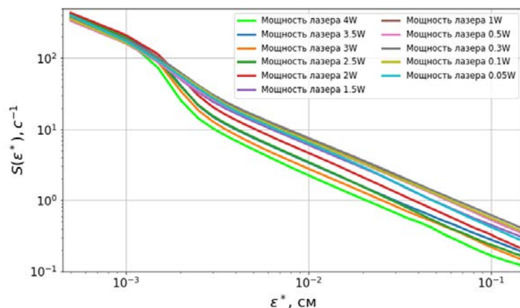
Рисунок 7. Динамические энтропии для мощности лазера от 4 Вт до 0.05 Вт.
