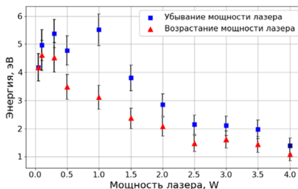
Рисунок 5. Кинетическая энергия при различных мощностях лазера.
