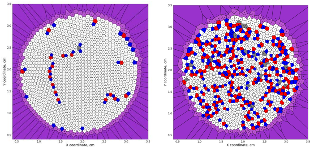
Рисунок 16. Диаграмма Вороного для структур, при воздействии лазерного излучения различной мощности а) 1 Вт, б) 4 Вт. Белым цветом отмечены частицы с шестью ближайшими соседями, фиолетовым цветом выделены периферийные частицы, синим и красным отмечены частицы с пятью и семью ближайшими частицами соответственно.
