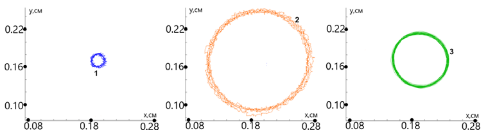
Рисунок 2. Траектории частиц за 8 секунд для 1 Вт. «1» голубым цветом отмечена пластиковая МФ-частица, «2» оранжевым - пластиковая частица с медной оболочкой, «3» зеленым – частица, частично покрытая медью (янус-частица).
