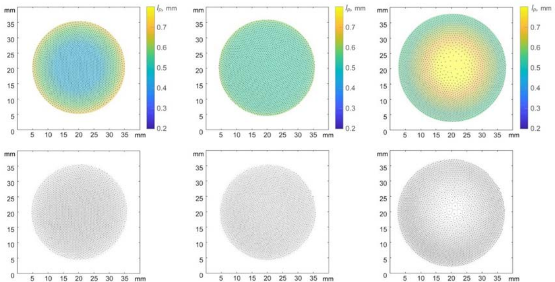
Рисунок 12. Квазидвумерная структура пылевых частиц в аргоновой плазме ВЧ разряда при мощности ВЧ разряда W=13.1 Вт и различной давлении буферного газа: а) 3 Па, б) 4 Па, в) 5 Па. На цветовой диаграмме приведено радиальное распределение межчастичного расстояния при различной мощности газового разряда. Снизу представлено изменение в однородности структуры - ячейки Вороного.
