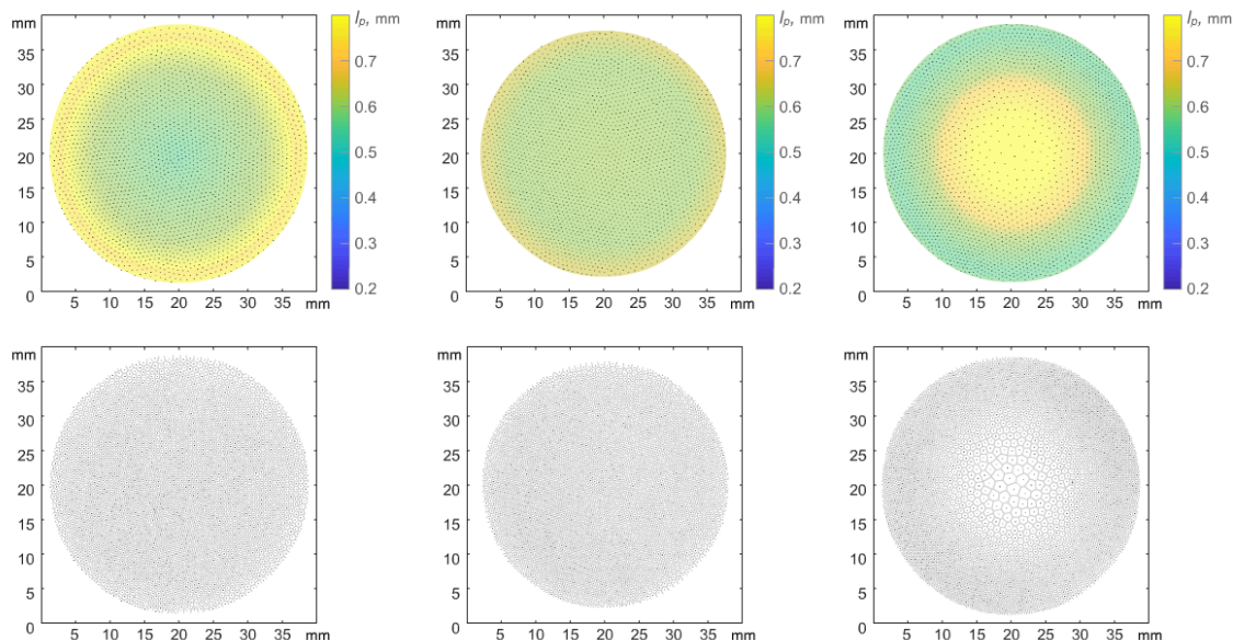
Рисунок 10. Квазидвумерная структура пылевых частиц в аргонной плазме ( p = 5 Па) при различной мощности ВЧ разряда: а) 4.4 Вт, б) 6.9 Вт, в) 16.7 Вт. На цветовой диаграмме приведено радиальное распределение межчастичного расстояния при различной мощности газового разряда. Снизу представлено изменение в однородности структуры - ячейки Вороного.
