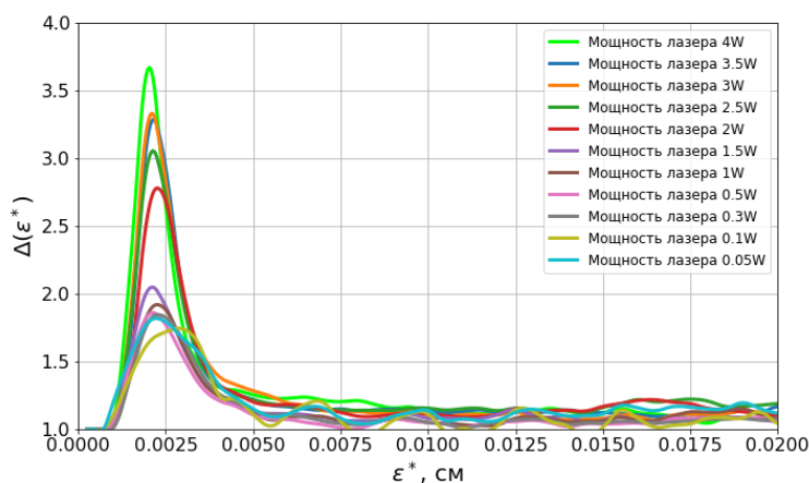
Рисунок 8. Функция фрактальной размерности для мощности лазера от 4 Вт до 0.05 Вт.
