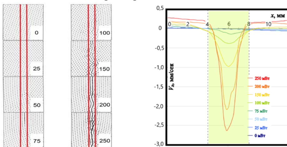
Рисунок 14. Траектории частиц и распределения скоростей при значениях мощности лазера W = 0; 25; 50; 75; 100; 150; 200 и 250 мВт. Область воздействия лазерного пучка отмечена зеленым цветом.
