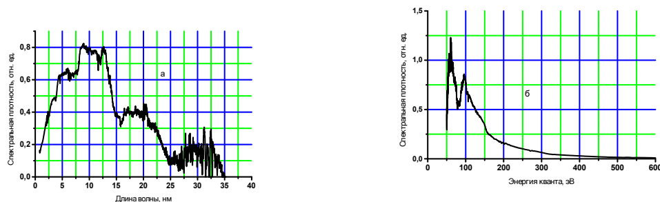
Рис.7. Спектр излучения вольфрамовой сборки: а – зависимость спектральной плотности излучения от длины волны; б – зависимость спектральной плотности излучения от энергии квантов. Ширина горизонтальной щели 700 мкм. Сборка – 80 проволок, диаметром 6 мкм, расположенных на диаметре 12 мм. Погонная масса сборки 440 мкг/см. Эксперимент № 4844.
