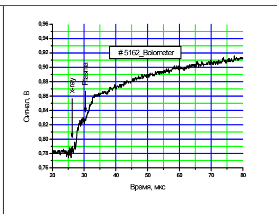
Рис.11. Сигнал радиационного калориметра при измерениях по направлению вдоль оси. Нагрузка 30 W проволочек диаметром 6 мкм на диаметре 20 мм. На аноде коллиматор диаметром 5 мм. Расстояние от пинча до фольги болометра 2.24 м. Стрелка указывает на момент излучения пинча.
