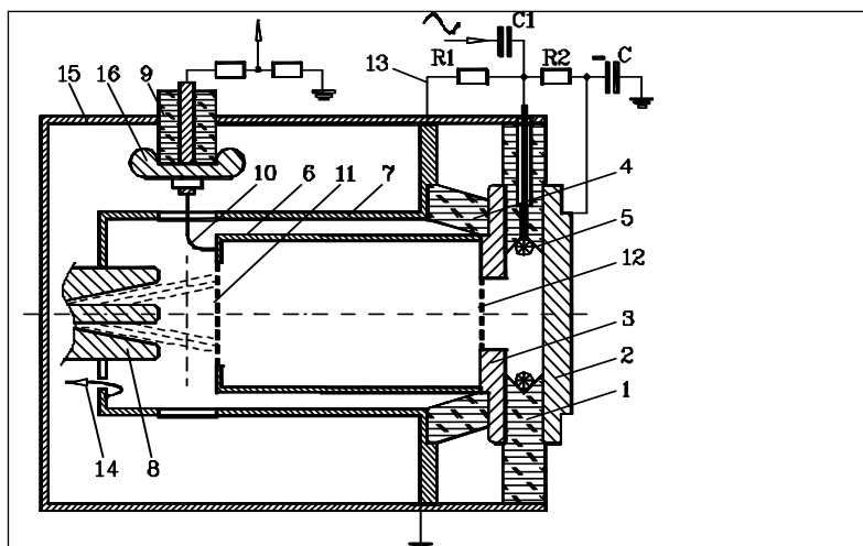
Рис.1 Схема установки. 1- корпус разрядника батареи; 2,3- электроды разрядника; 4-входной вакуумный изолятор; 5-поджигающий электрод разрядника; 6 -катодный коаксиал; 7 - анодный коаксиал; 8 – газовое сопло; 9-высоковольтный омический делитель напряжения; 10- вывод напряжения с катодного коаксиала; 11,12 – металлические сетки; 13- высоковольтный делитель; 14 - магнитная петля; 15-корпус вакуумной камеры; 16- экранирующий электрод высоковольтного делителя напряжения.
