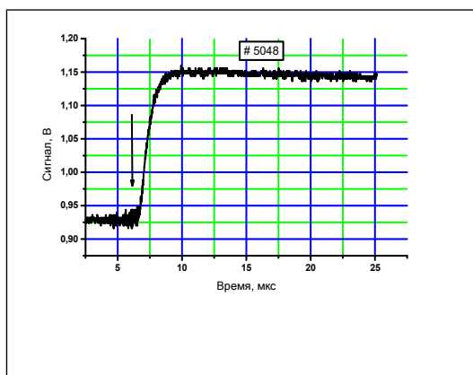
Рис.10 Сигнал радиационного калориметра. Направление измерений – сбоку по отношению к оси лайнера. Нагрузка 40 W диаметром 6 мкм, 220 мкг/см, диаметр сборки 12 мм. Расстояние от пинча до чувствительного элемента болометра 2.24 м. Стрелка указывает на момент излучения пинча.
