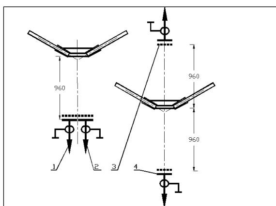
Рис.5. Схема экспериментов по исследованию излучения 16-ти канального разряда с помощью ВУФ датчиков. 1 – фильтрованный датчик, фильтр - цапонлак 7.8 \text{ мкг/см}^2 . 2,3,4 – открытые ВУФ датчики.
