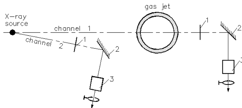
Рис.2.22. Схема просвечивания струи мягким рентгеновским излучением: 1 - рентгеновские фильтры, 2 - тонкие сцинтилляторы, 3 - фотоумножители.
