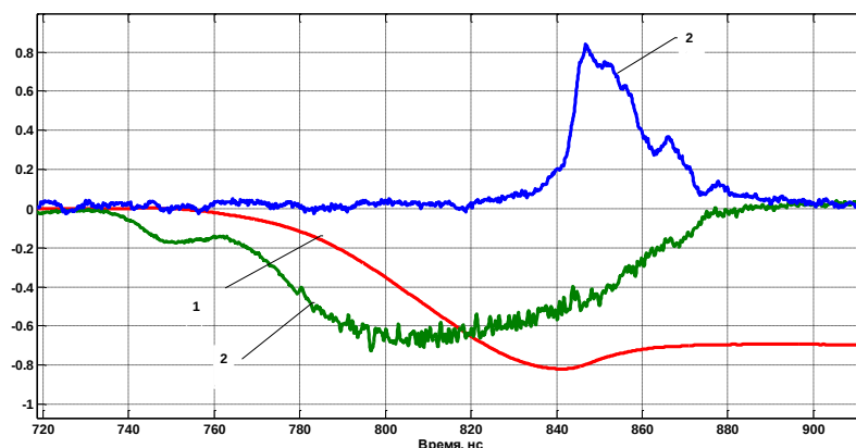
Рис. 6.16. Осциллограммы сигналов полученные при сжатии каскадной нагрузки: 1 - ток через нагрузку /5Е6 (Ампер); 2 - напряжение на нагрузке/1Е6(Вольт); 3 -сигнал ВРД s2e/2Е1 (Вольт). Каскадная нагрузка. Внешняя сборка 40 алюминиевых проволок диаметром 18 мкм ( m_{п}=275 мкг/см) на диаметре 12 мм, внутренняя сборка 6 вольфрамовых проволок диаметром 6мкм ( m_{п}=32 мкг/см) на диаметре 5 мм.
