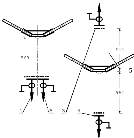
Рис.5.17. Схема экспериментов по исследованию излучения 16-ти канального разряда с помощью ВУФ датчиков. 1 – фильтрованный датчик, фильтр – нитроцеллюлоза 7.8 \text{ мкг/см}^2 . 2,3,4 – открытые ВУФ датчики, 5 – кабели РК-50-9-13.
