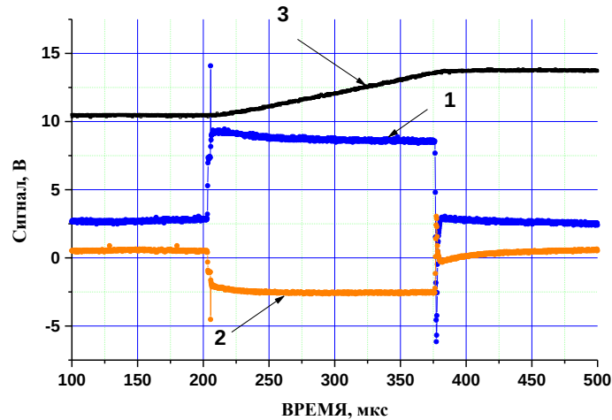
Рис.1.9. Калибровка чувствительности радиационного калориметра: 1 – сигнал напряжения на фольге при дополнительном подогреве, 2 – сигнал тока дополнительного подогрева (увеличен в 5 раз), 3 – калибровочный сигнал с фотодетектора (увеличен в 50 раз). Длительность калибровочного импульса дополнительного подогрева 170 мкс.
