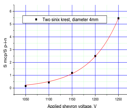
Рис.2.13(б) Зависимость чувствительности МКП детектора шевронного типа от величины приложенного напряжения. Диаметр чувствительной области 4 мм. Красная кривая – подгонка экспоненциальной зависимостью.
