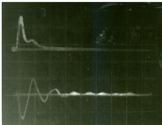
Рис.5.9(а). Разряд по флешбоду: Верхняя осциллограмма -- сигнал фотодиода закрытого фильтром цапонлак 13 мкг/см 2 ( S = 1.5 см 2 ), 0.05 В/дел. Нижний сигнал -- ток разряда, по горизонтали 2 мкс/дел
