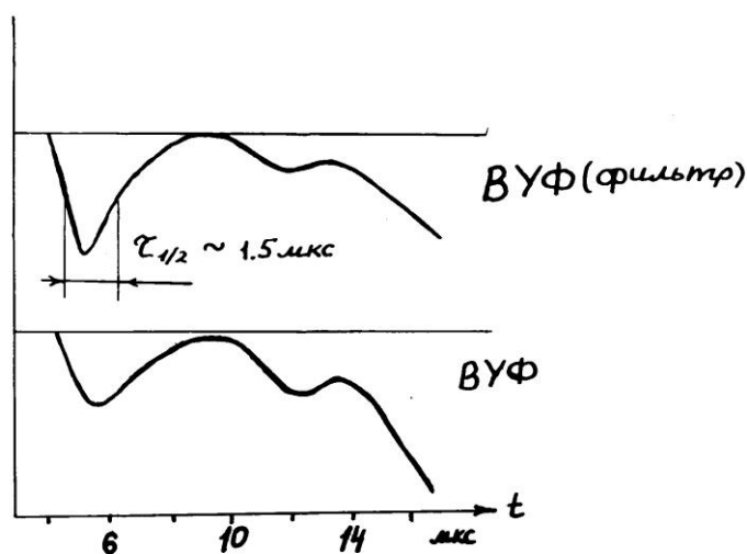
Рис.5.21. Многоканальный разряд в вакууме. Повреждение фильтра плазмой.
