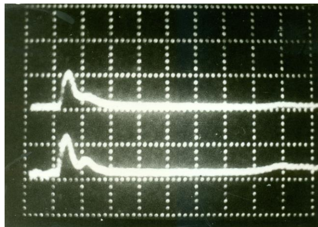
Рис.5.9(б). Разряд по флешбоду: Верхняя осциллограмма --- сигнал фотодиода закрытого фильтром цапонлак 13 мкг/см 2 ( S = 1.5 см 2 ) 0.1 В/дел. Нижний сигнал --- сигнал открытого фотодиода ( S = 0.44 см 2 ), 5 В/дел. по горизонтали 2 мкс/дел
