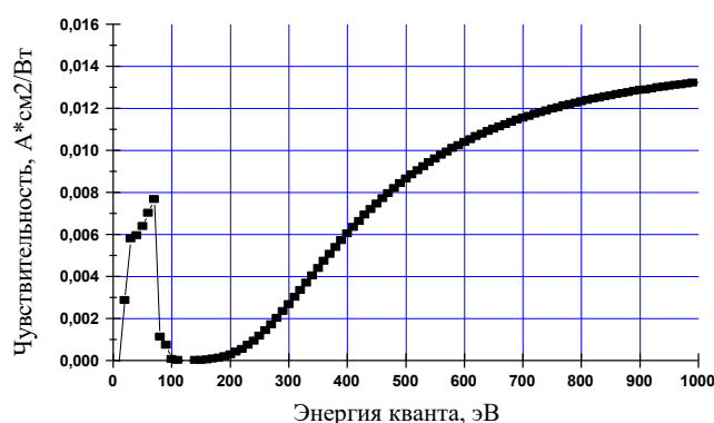
Рис.2.16. Расчетная спектральная чувствительность кремниевого детектора СППД–11-04 от энергии кванта (чувствительная область детектора \delta = 80 мкм, алюминиевое контактное покрытие 0.1 мкм, “мертвый слой” кремния 0.15 мкм).
