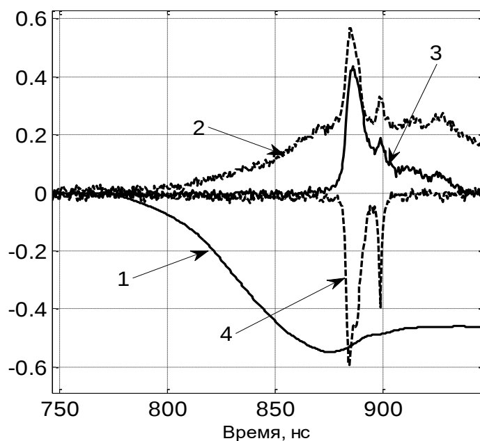
Рис.4.4. Эксперимент № 4859 1– ток пинча, I_{\text{max}} = 2.8 \text{ МА} , 2 - сигнал ВРД-датчика s3e ( h\nu > 20 \text{ эВ} ), 3 -сигнал ВРД-датчика s2e ( h\nu > 130 \text{ эВ} ), 4 - сигнал ВРД-датчика s4e ( h\nu > 700 \text{ эВ} ).
