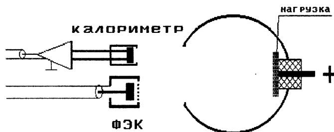
Рис.5.5. Схема экспериментов по исследованию пробоя по поверхности диэлектрика в воздухе.
