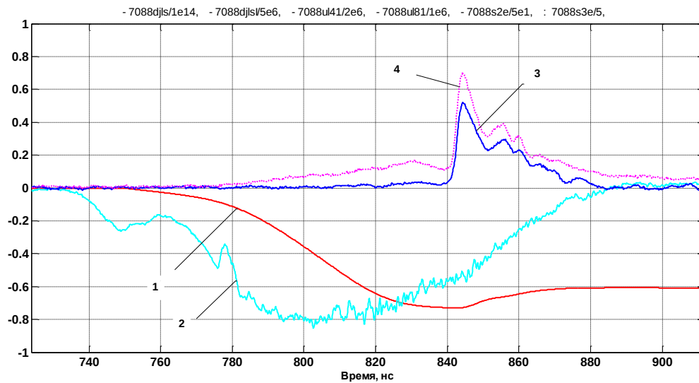
Рис.8.15. Эксп. № 7088. Синхронизованные осциллограммы сигналов рентгеновского излучения, напряжения и тока. 1- ток I через пинч I/5e6 (A); 2 - напряжение U на пинче U/1e6 (B); 3- сигнал с вакуумного рентгеновского диода s2e/5e1 (B) ( h\nu > 130 эВ); 4 - сигнал с вакуумного рентгеновского диода s3e/5 ( h\nu > 30 эВ) (B).
