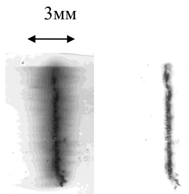
Рис. 7.12. Эксперимент № 4847. Обскурограмма пинча, снятая в квантах с энергией свыше 150 эВ (слева) и свыше 600 эВ (справа).
