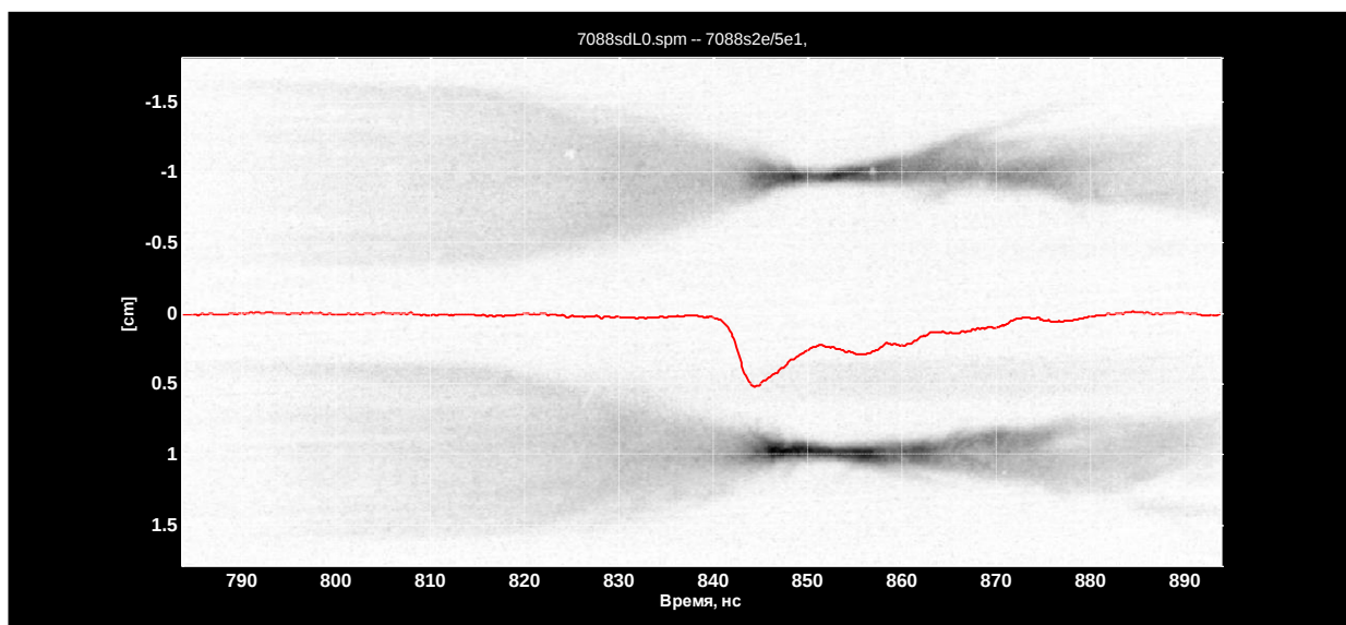
Рис.8.16. Эксп. № 7088 Радиальные оптические щелевые развертки с наложенным на них синхронизованным сигналом мягкого рентгеновского излучения ВРД s2e/5e1 (B) ( h\nu \geq 150 эВ).
