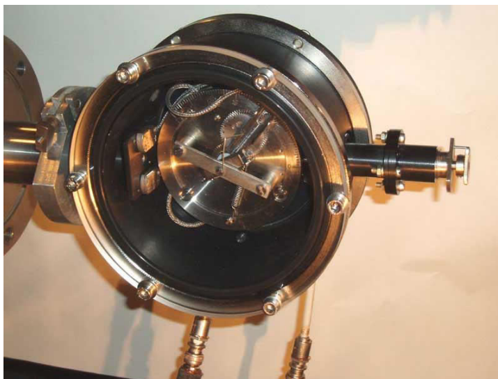
Рис.2.14. Внешний вид спектрометра СМНР-4.
