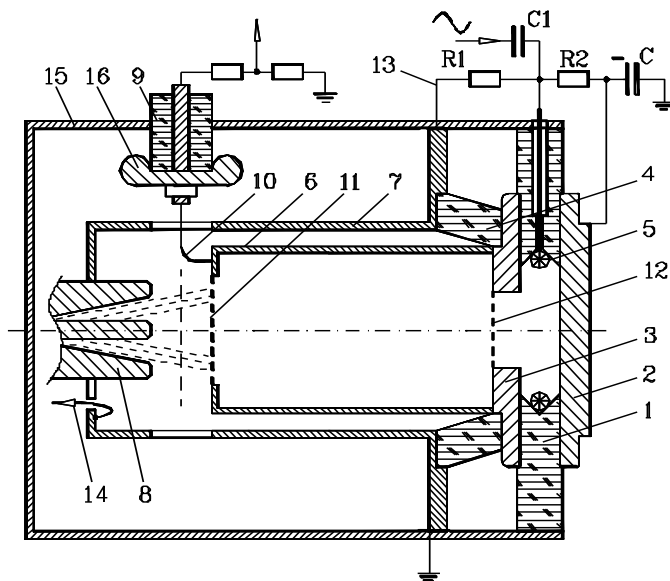
Рис.2.1 Схема установки.
