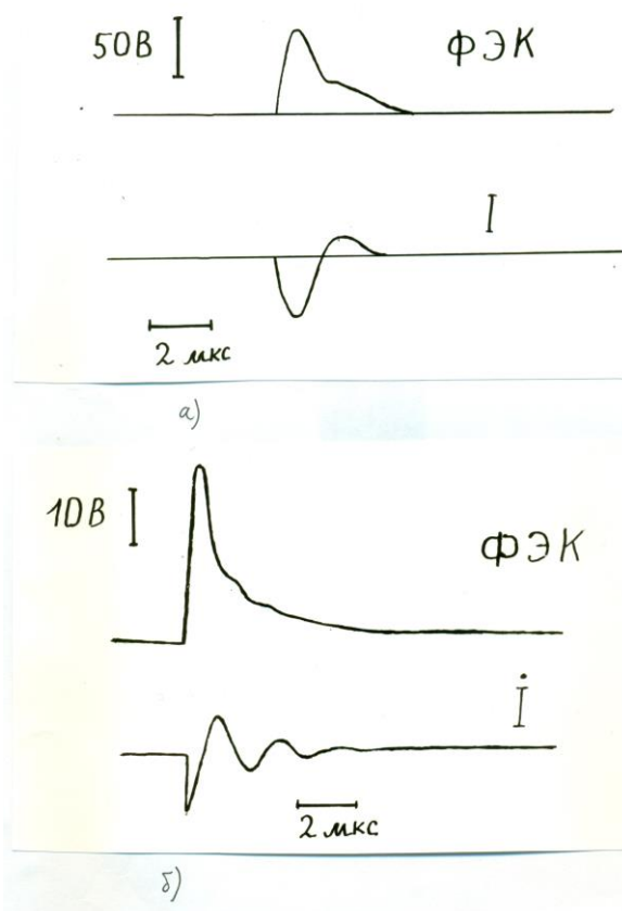
Рис.5.7. Характерные осциллограммы:
