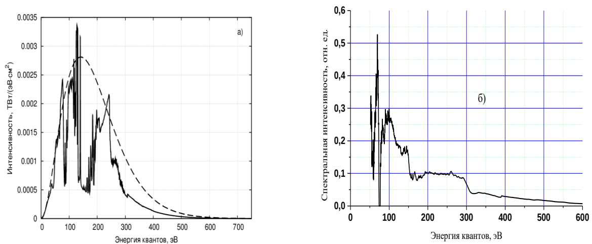
Рис. 6.9 Сравнение расчетного спектра излучения однородного цилиндрического столба плазмы вольфрама радиуса R = 0.1 см при плотности электронов N_e = 10^{21} 1/см 3 и температуре T_e = 50 эВ с экспериментом 4847. а - расчетный спектр, штриховая кривая – спектр черного тела при температуре 50 эВ; б – спектр, полученный в эксперименте № 4847.
