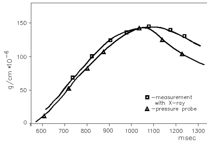
Рис.2.24. Зависимость погонной массы струи от времени при давлении в клапане 4 атм. Не профилированное сопло с числом Маха M = 2 .
