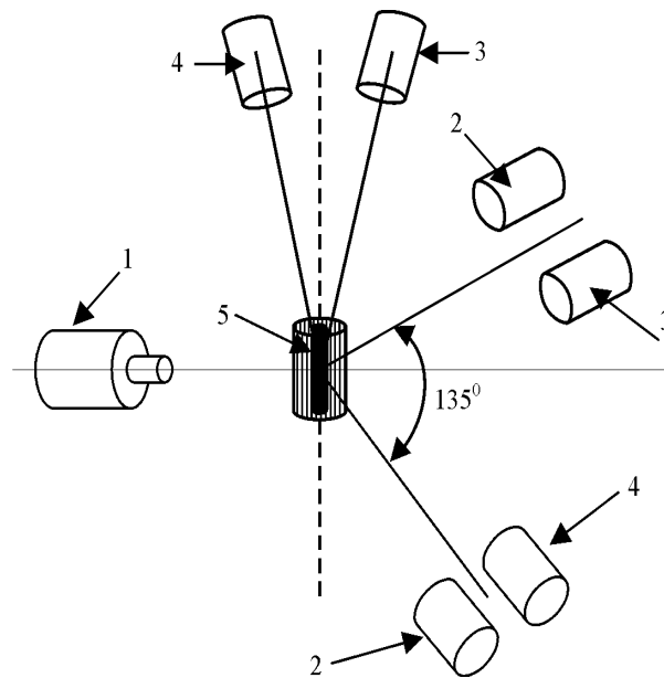
Рис.7.1. Схема расположения диагностических методик: 1- камера обскуры, 2 – термопарные калориметры, 3 - ВРД с фильтрами, 4 - болометр, 5 - пинч. Направление наблюдения – сбоку относительно оси пинча.
