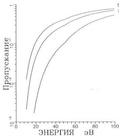
Рис.5.12. Пропускание фильтров из нитроцеллюлозы с поверхностными массами 5, 7, 13 мкг/см 2 .
