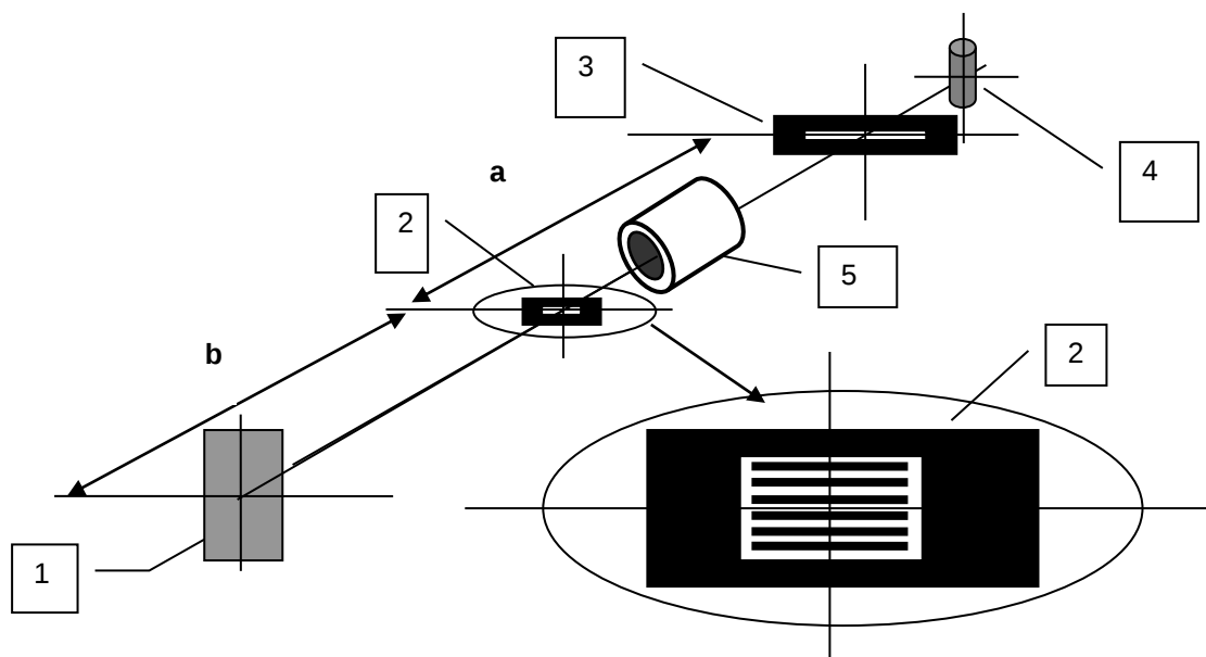
Рис.1.13. Геометрия схемы спектрографа с пропускающей решеткой. 1- рентгеновская пленка, 2 – блок с пропускающей решеткой (штрихи решетки параллельны спектральной щели), 3 - спектральная щель, 4 – пинч, 5 – электромагнитный шторный затвор.
