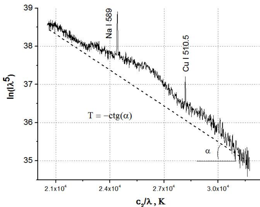
Рис. 4.3.4.3. Спектр периода послесвечения t_{\text{имп}} + (5 \div 7) мс в координатах Вина. T \sim 3000\text{K}
