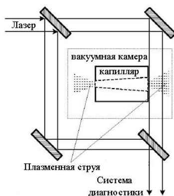
Рис. 1.1.4.2. Схема регистрации данных. D. Kaganovich и др. [60]
