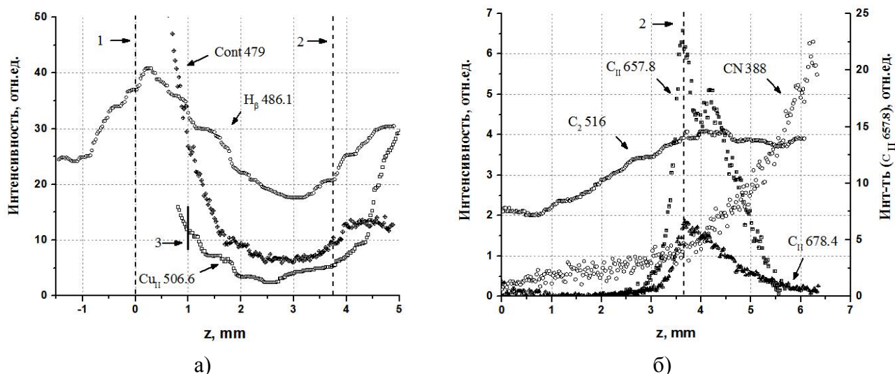
Рис. 4.2.3.3. Продольный ход интенсивности H \beta , Cu II и континуума (а) и C II, C 2 и CN (б). 1 – граница капилляра, 2 – центральный скачок уплотнения. Сверхзвук, середина импульса, 3 – граница слияния сильно уширенных спектральных линий Cu II с континуумом
