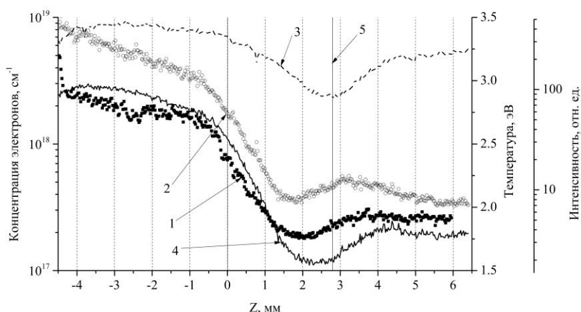
Рис. 4.2.3.6. Параметры плазмы вдоль оси струи: (1) - электронная концентрация, (2) - электронная температура, (3) - интенсивность излучения линии H_{\alpha} , (4) - интенсивность непрерывного излучения на длине волны \lambda=672 нм, (5) – положение диска Маха ( Z \approx 2.8 мм). Сечение z=0 соответствует положению среза капилляра.
