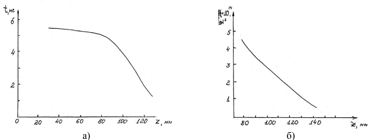
Рис. 1.1.2.3. Время существования концентрации электронов, превышающей критическую n_{кр} = 1.6 \cdot 10^{13} , в зависимости от расстояния от сопла плазматрона (а) и максимальное значение концентрации электронов вдоль оси струи (б). МГУ [46]
