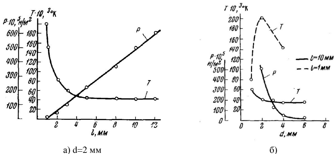
Рис. 1.1.1.2. Зависимость температуры и давления плазмы внутри капилляра от длины (а) и диаметра (б) капилляра. I = 9000 А. Н.Н. Огурцова, И.В. Подмошенский, В.М. Шеленина [54]
