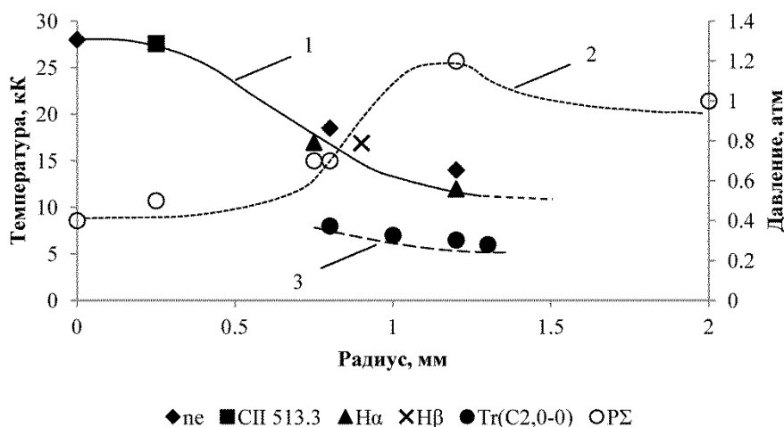
Рис. 4.2.4.2. Распределение параметров плазмы в сечении z=2.5 мм: 1 – температура электронов, 2 – давление, 3 – вращательная температура T_r (полоса (0-0) радикала C 2 ).
