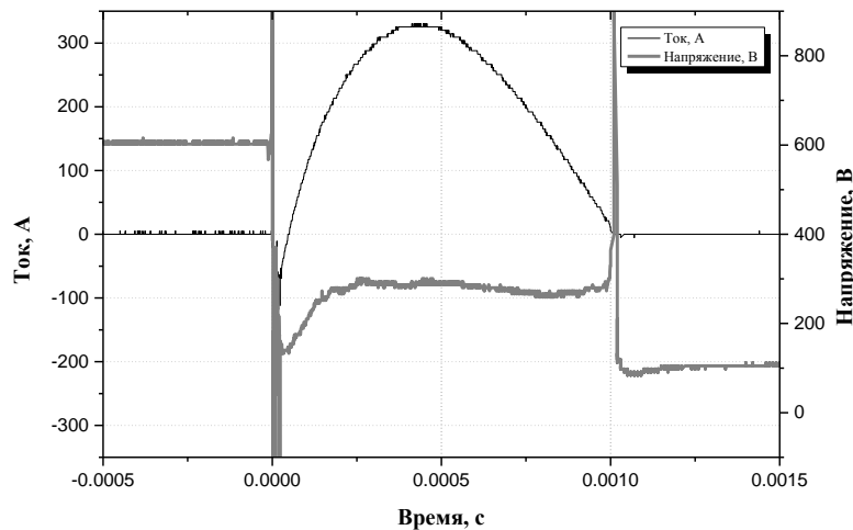
Рис. 2.1.2.3. Осциллограмма разряда в сверхзвуковом режиме истечения
