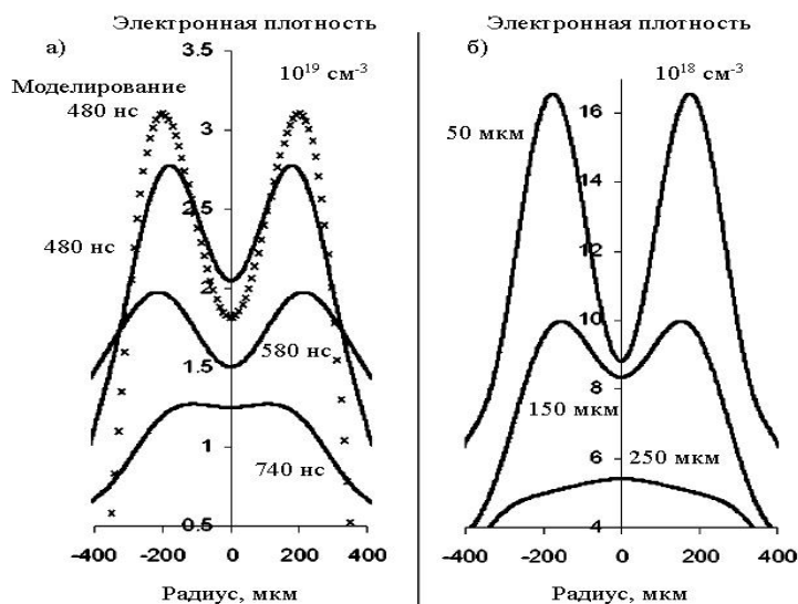
Рис. 1.1.4.3. Распределения электронной плотности плазмы во времени (а) на расстоянии 50 мкм от среза широкой части (0.5 мм) капилляра и в пространстве (б) через 600 нс после инициализации разряда. Точками показано расчётное распределение в модели D. Kaganovich и др. [60]
