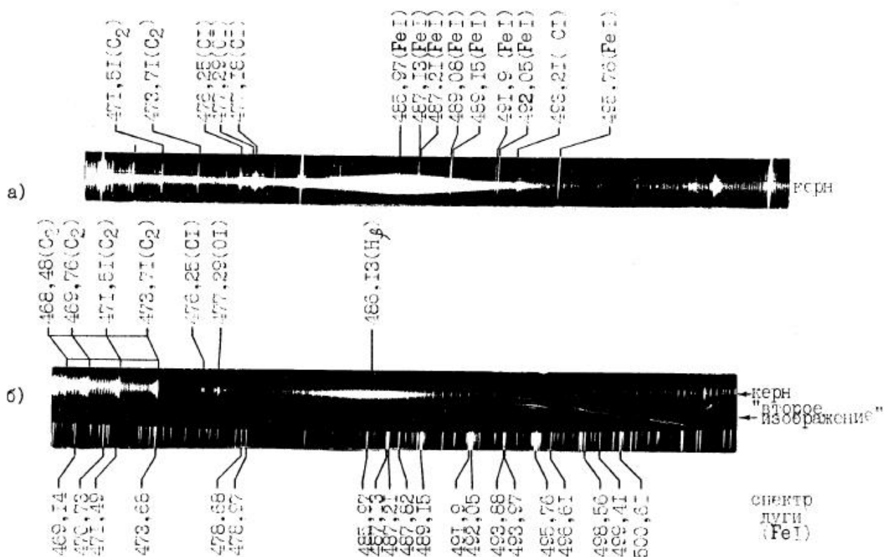
Рис. 1.1.3.3. Спектр факела с широким (а) и узким (б) керном (область Н β ). МИФИ [49]
