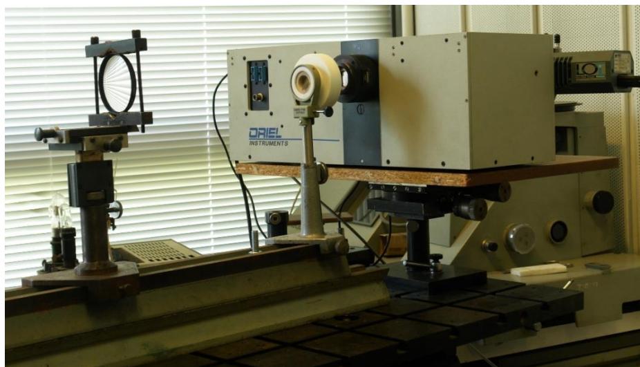
Рис. 2.2.4.1. Общий вид спектрометра MS-257 с фокусирующим конденсором и призмой Дове.
