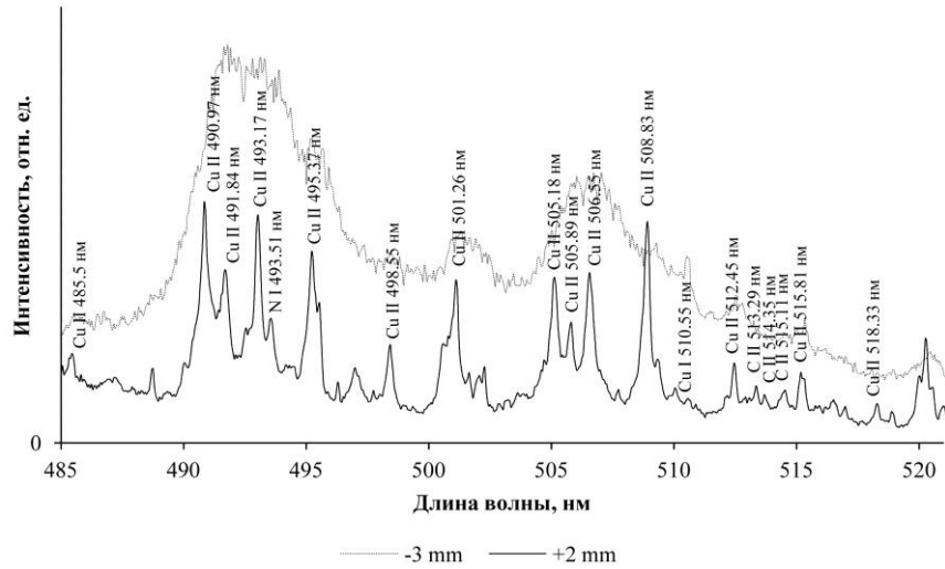
Рис. 2.3.7.3. Детальные спектры излучения плазмы внутри капилляра ( z=-3 мм) и на начальном участке струи ( z=+2 мм). В скобках указаны расстояния от среза капилляра. MS-257. Длительность экспозиции камеры спектрографа 5 мкс.
