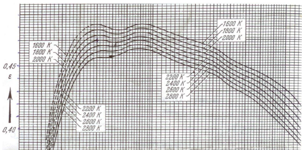
Рис. 2.2.7.1. Коэффициент излучения эталонной ленточной лампы накаливания
