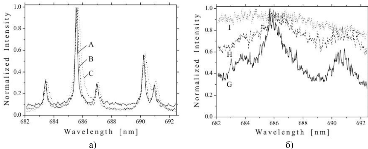
Рис. 1.1.5.3. Уширение спектральных линий фтора при энерговкладах А – 10 Дж·см ^{-3} , В – 20 Дж·см ^{-3} , С – 30 Дж·см ^{-3} (а) и при энерговкладах G – 7.5 кДж·см ^{-3} , H – 10 кДж·см ^{-3} , I – 12.5 кДж·см ^{-3} (б). S.Kukhlevsky, J. Kaiser, O. Samek и др. [64]
