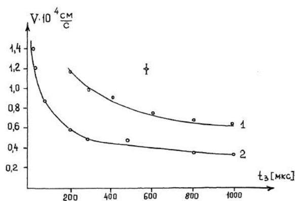
Рис. 1.1.3.2. Зависимость скорости распространения лазерного факела от времени. 1) d=1 мм, 2) d=2 мм. МИФИ [49]
