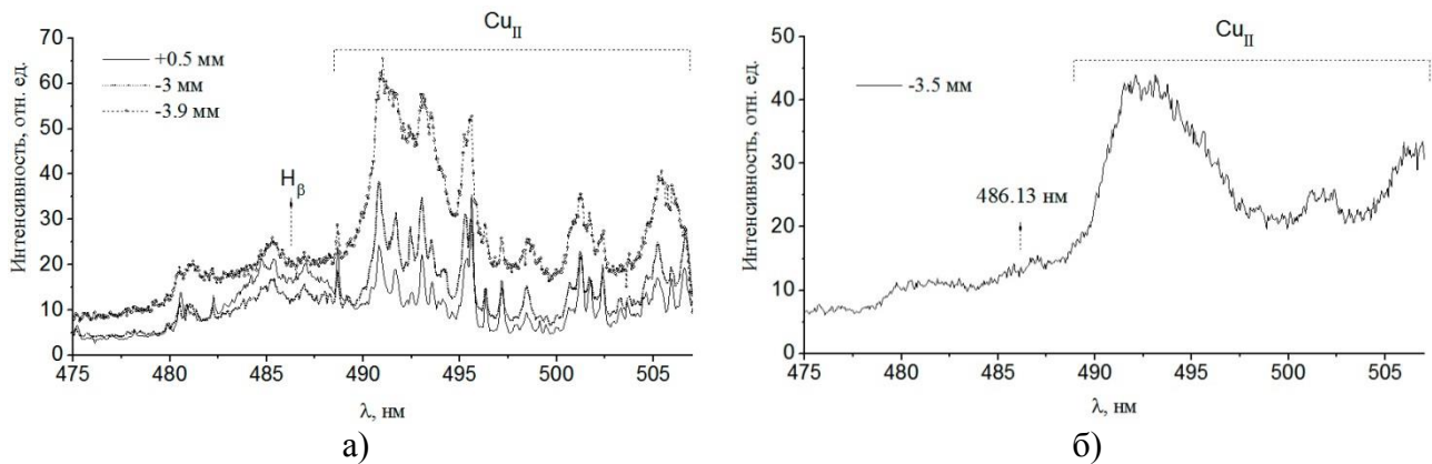
Рис. 2.3.7.4. Спектры излучения в диапазоне 475 \div 505 нм внутри капилляра при продольной регистрации на разных высотах (а) и при поперечной регистрации в центре (б). Сверхзвуковой режим истечения струи. Момент времени - 500 мкс. Координаты регистрации указаны относительно среза капилляра. Экспозиция кадра – 40 мкс.
