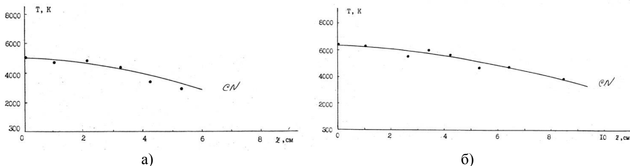
Рис. 1.1.2.5. Зависимость температуры плазмы от продольной координаты z при W = 100 Дж (а) и W = 200 Дж (б) . МГУ [46]
