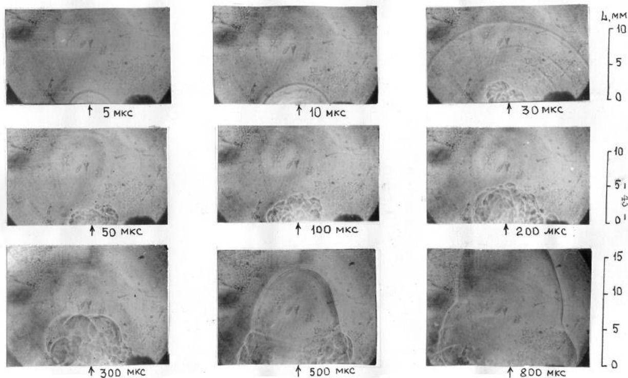
Рис. 1.1.3.1. Теневые фотографии начальной стадии формирования факела. МИФИ [49]
