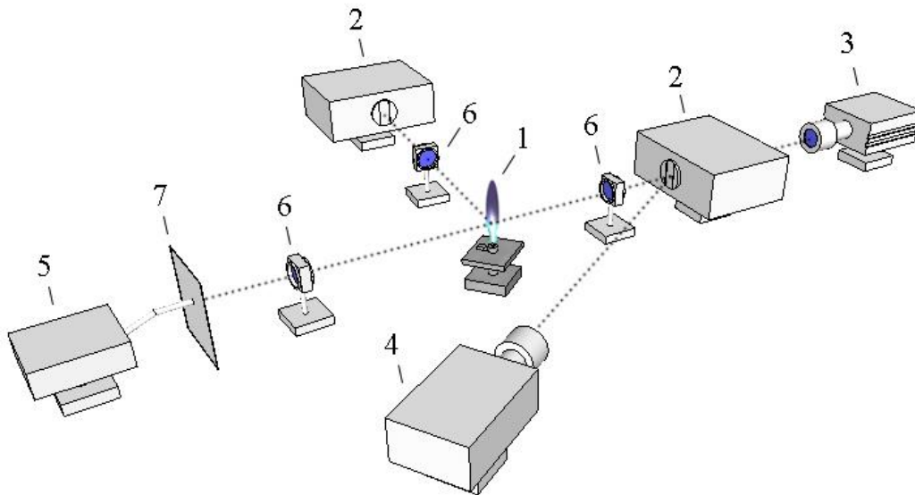
Рис. 2.2.3.1. Система оптических измерений параметров эрозионной плазменной струи. 1 – исследуемый объект, 2 – спектрограф Oriol MS-257, 3 – камера Andor/Andor iStar DH720/VS Fast, 4 – камера MotionPro, 5 – спектрограф AvaSpec 2048, 6 – кварцевая линза, 7 – экран с масштабной сеткой
