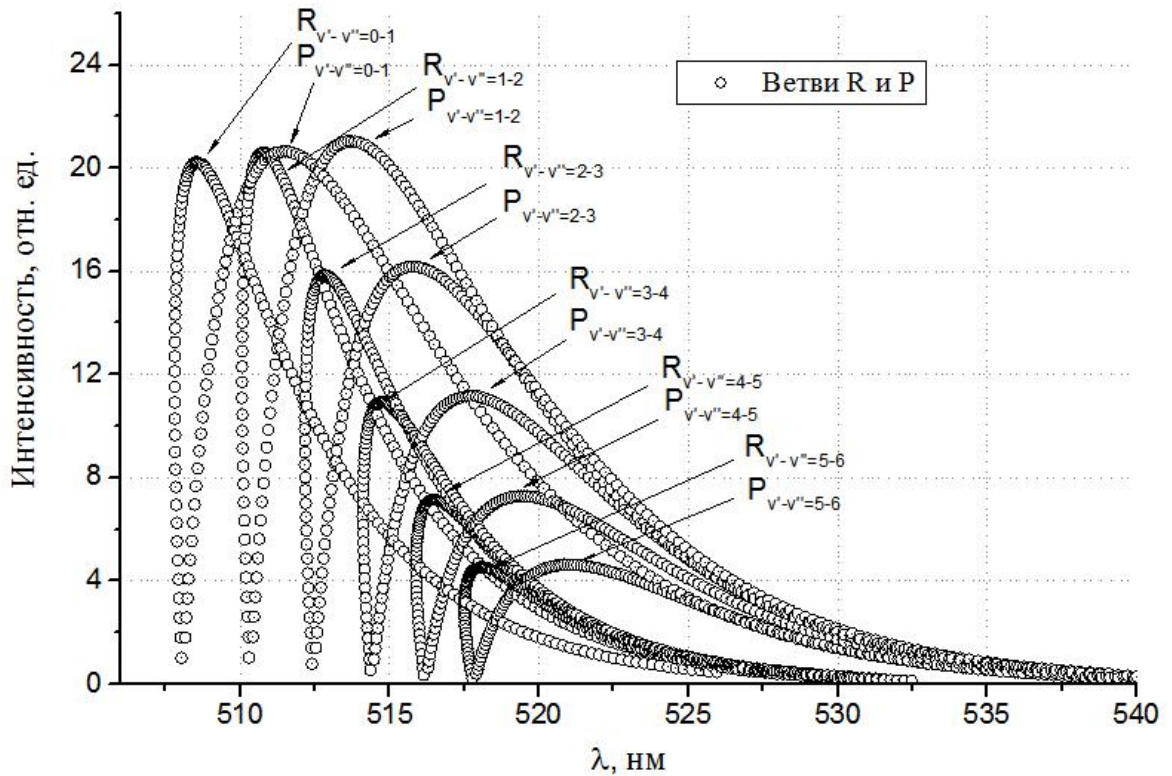
Рис. 3.4.8.3. Модель вращательных ветвей R и P колебательных переходов v'-v''=0-1, 1-2, 2-3 \dots электронного перехода B^2\Sigma^+ - X^2\Sigma^+ молекулы AlO. Вращательная и колебательная температуры равны T_v = T_r = 0.3 эВ
