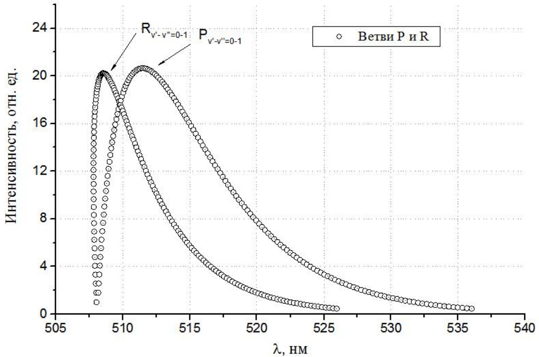
Рис. 3.4.8.2. Модель вращательных ветвей R и P колебательного перехода v'-v''=0-1 в электронном переходе V^2\Sigma^+ - X^2\Sigma^+ молекулы \text{AlO} . Вращательная температура T_r = 0.3 эВ
