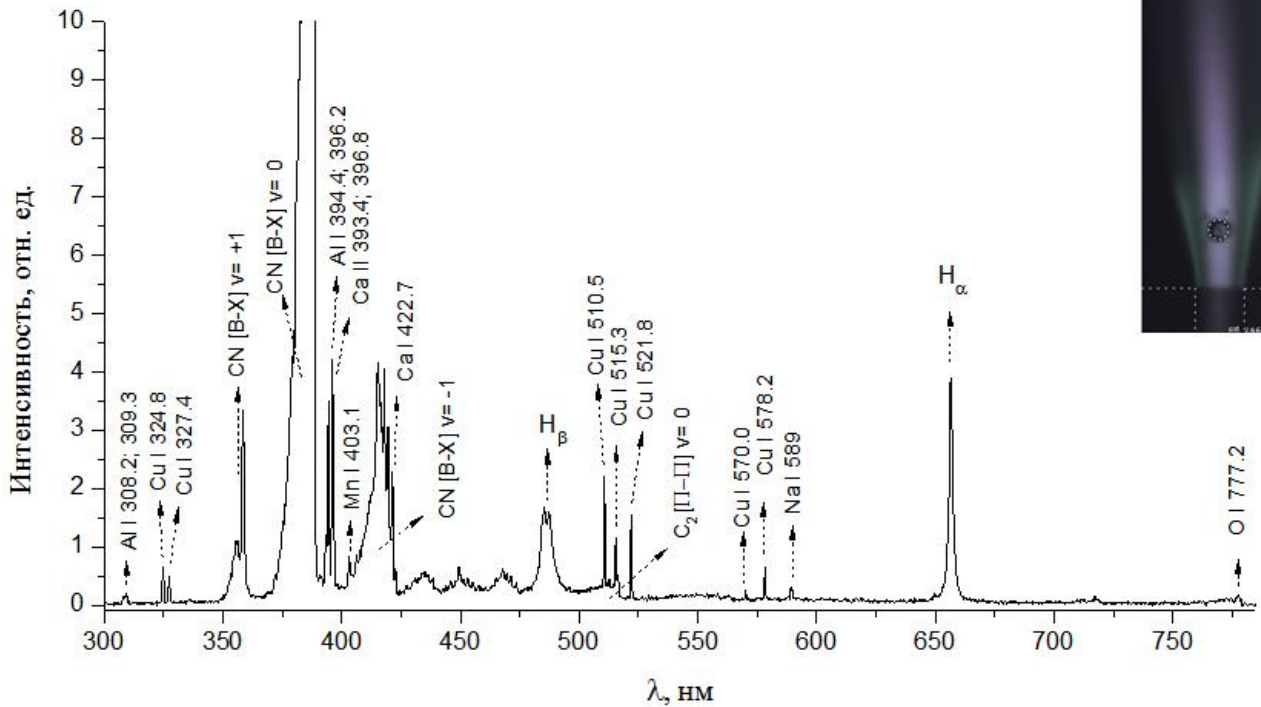
Рис. 2.3.7.1. Спектр излучения на начальном участке струи ( h=3.5 мм от среза капилляра).
