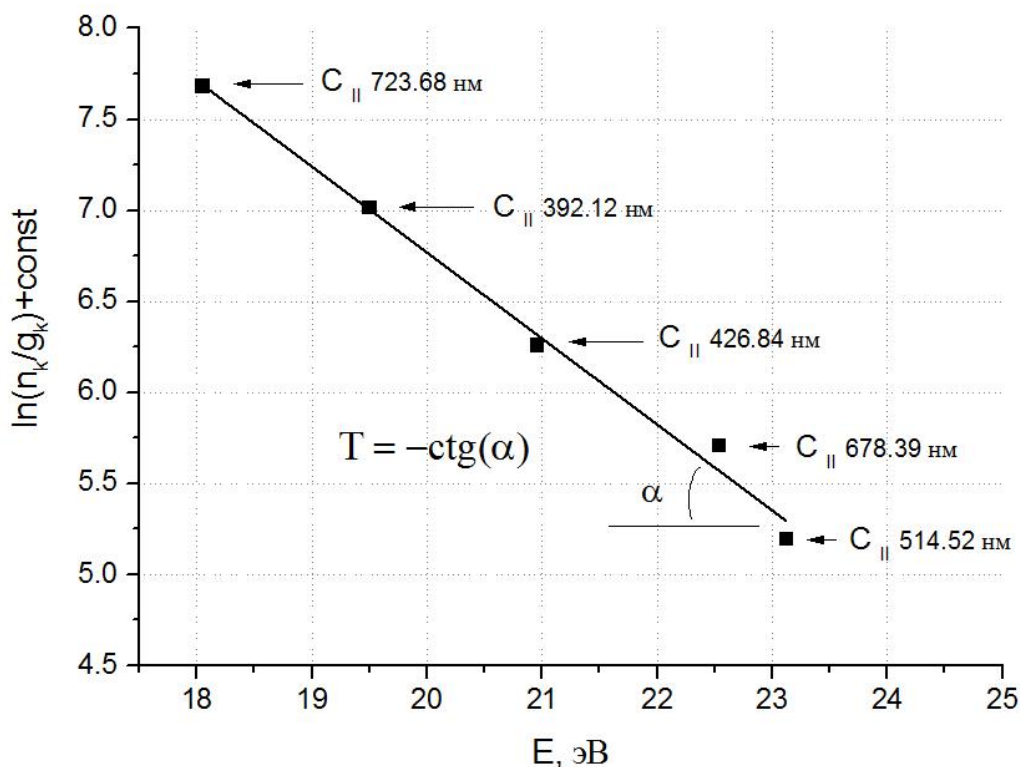
Рис. 3.3.5.3. «Больцмановская экспонента» заселённости ионов углерода в сверхзвуковом режиме истечения струи. T = 2.12 \pm 0.34 эВ, h = 2 мм, \tau = -1.5-0.5 мс
