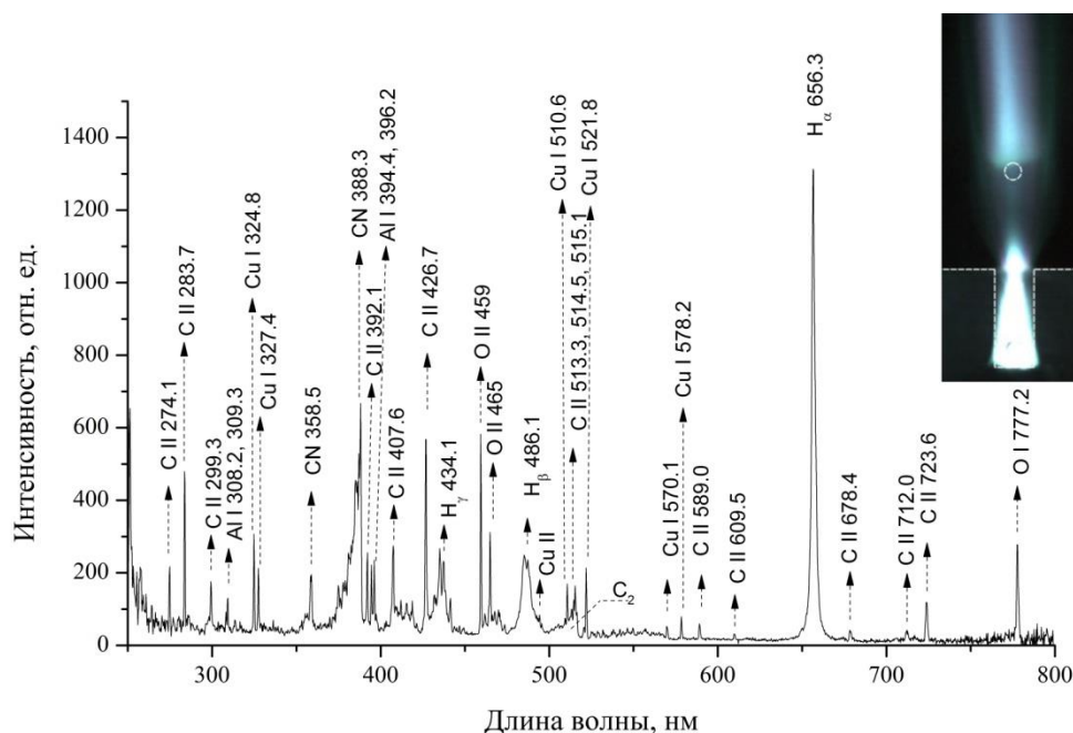
Рис. 2.3.7.2. Спектр излучения на начальном участке струи ( h=3.0 мм от среза капилляра).
