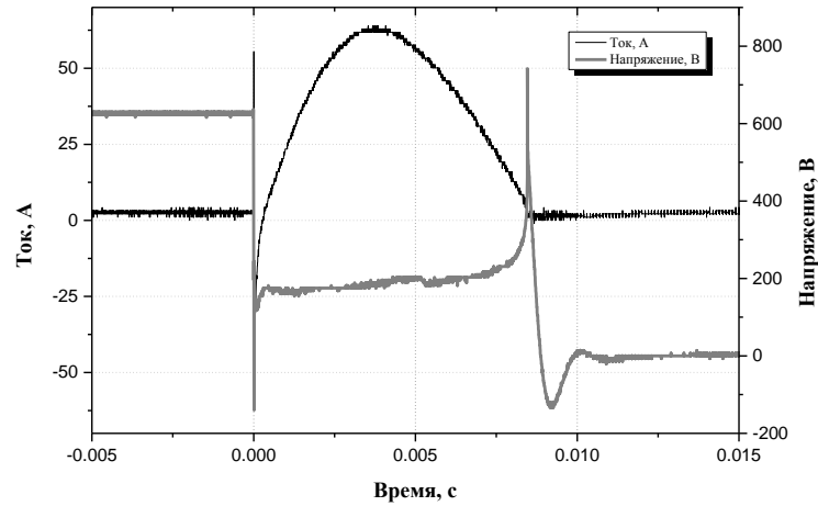
Рис. 2.1.2.2. Осциллограмма разряда в дозвуковом режиме истечения
