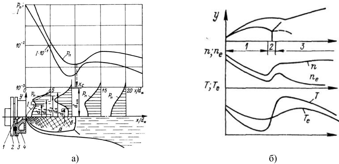
Рис. 4.2.3.2. Схема течения на начальном участке недорасширенной затопленной струи плазмы аргона, истекающей из звукового сопла электродугового источника (а).
